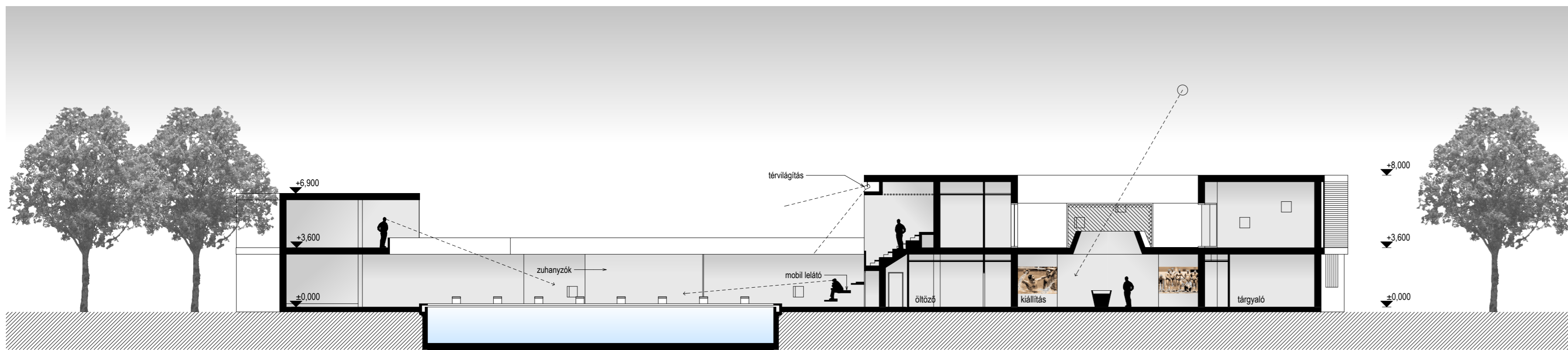
C-C metszet
