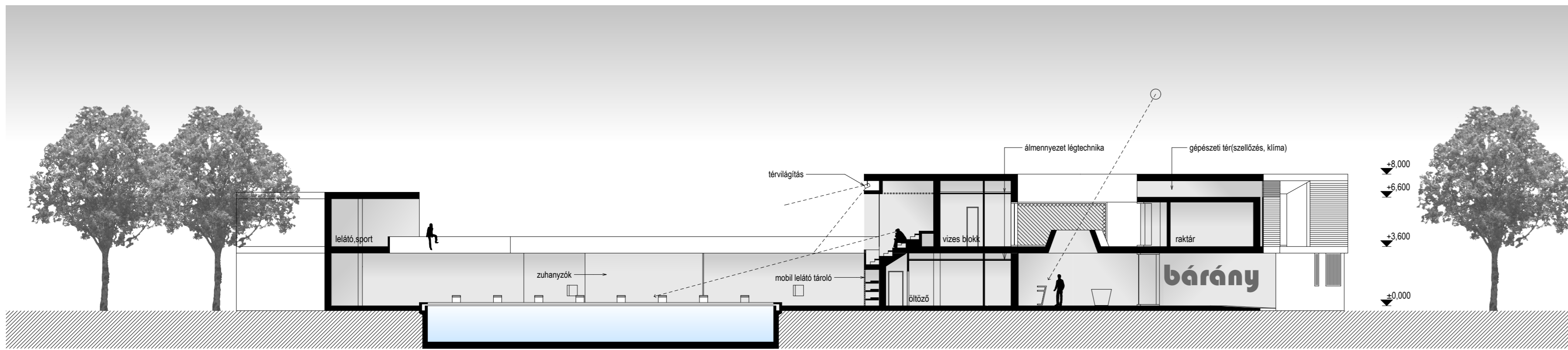
B-B metszet
