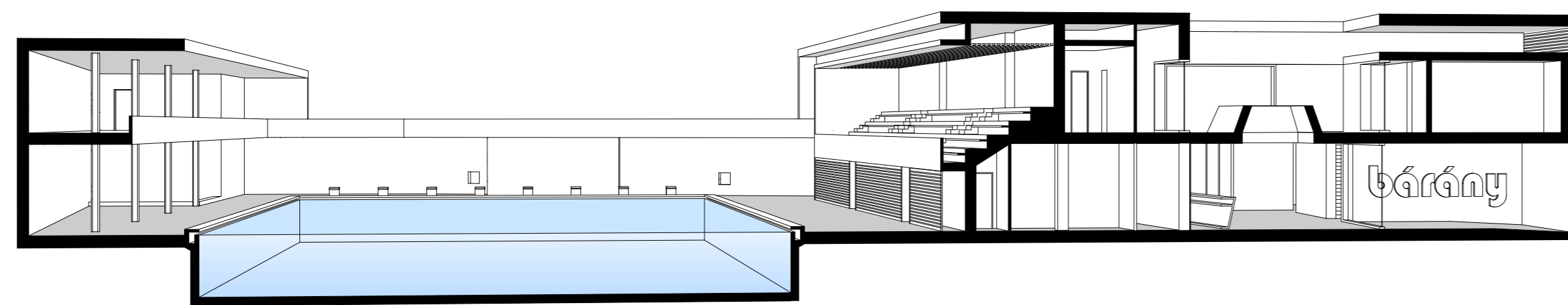
Térbeli keresztmetszet
