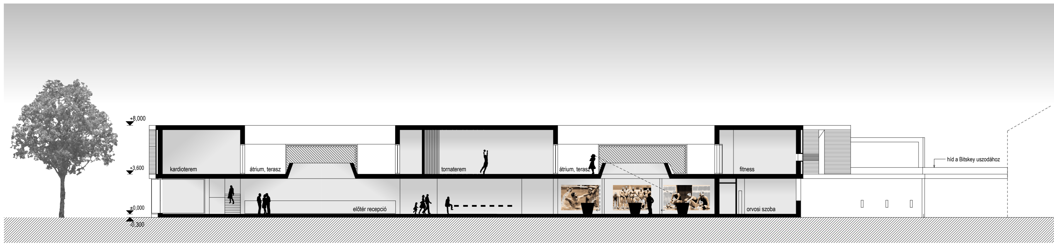
A-A metszet
