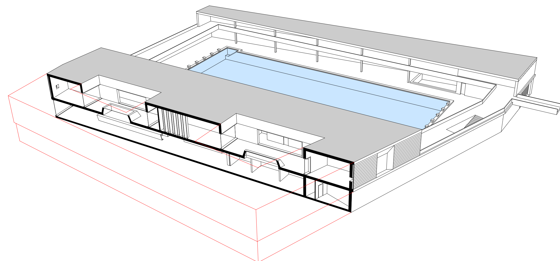
Térbeli metszet a fejépületen keresztül
