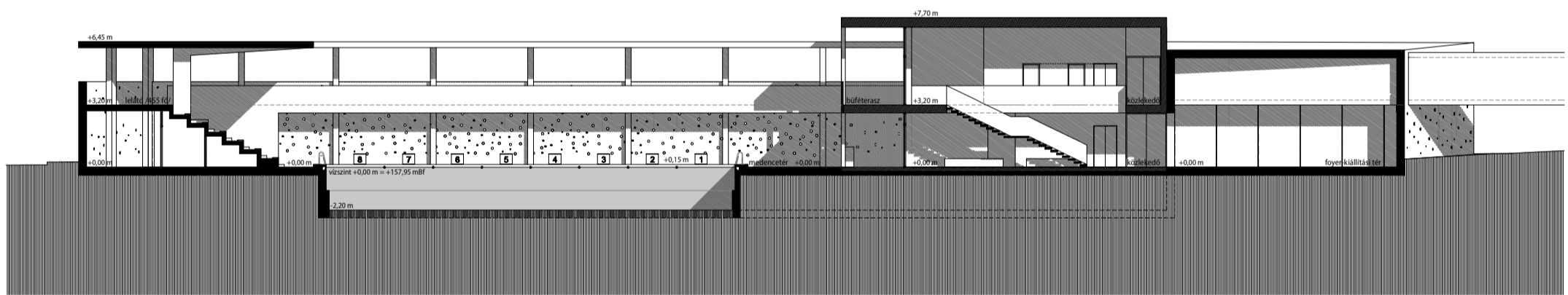
metszet a medencén keresztül m=1:200
