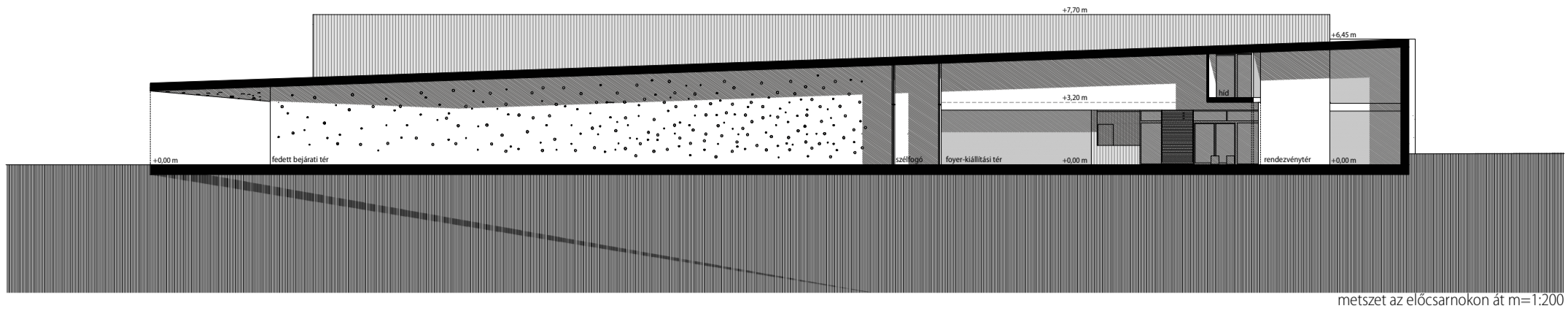
metszet az előcsarnokon át m=1:200
