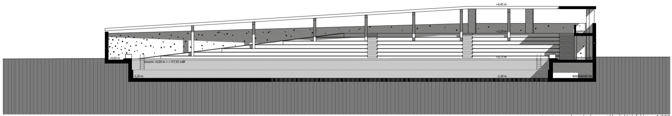
metszet a medencén keresztül a lelátó felé m=1:200
