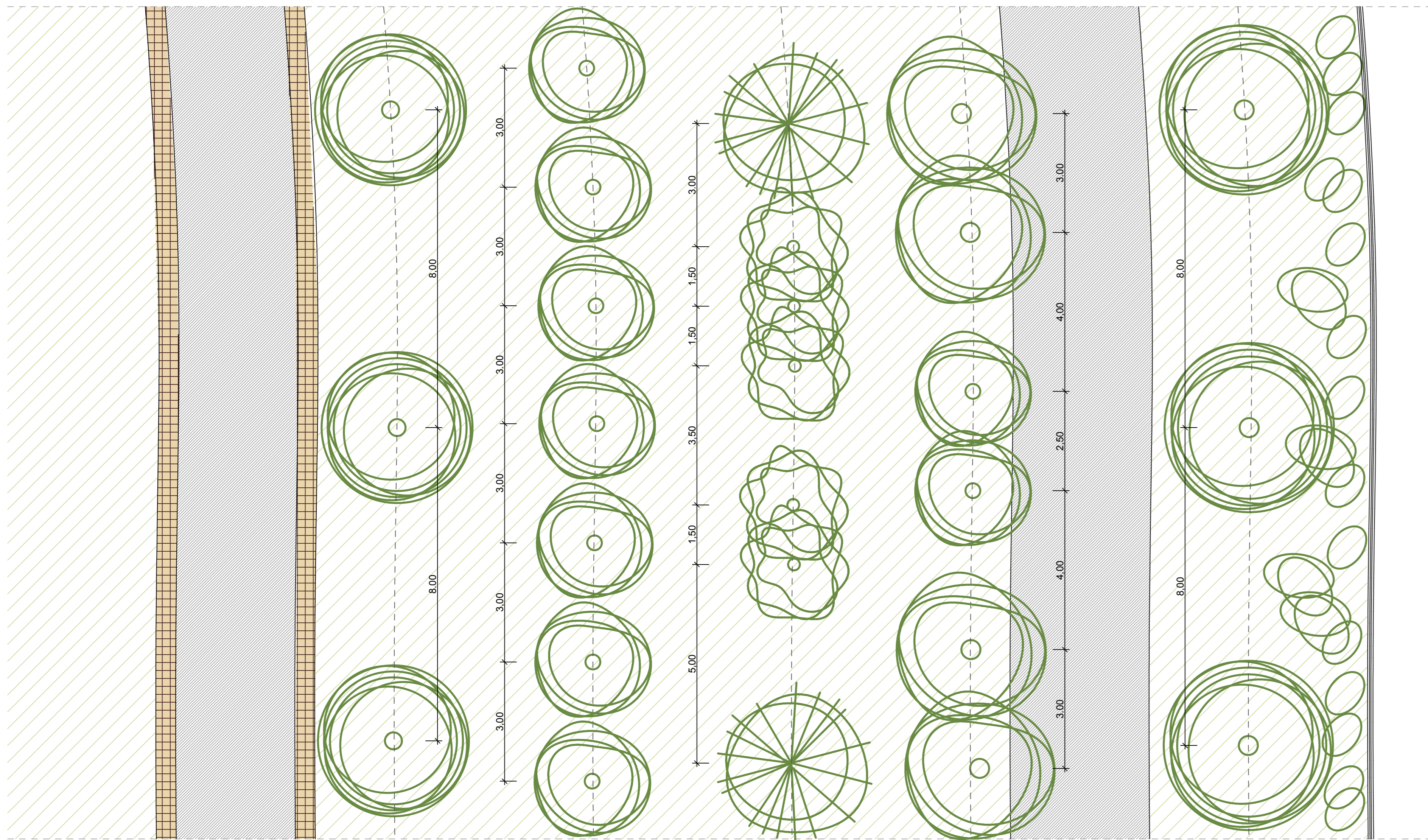
Alaprajz M=1:100
