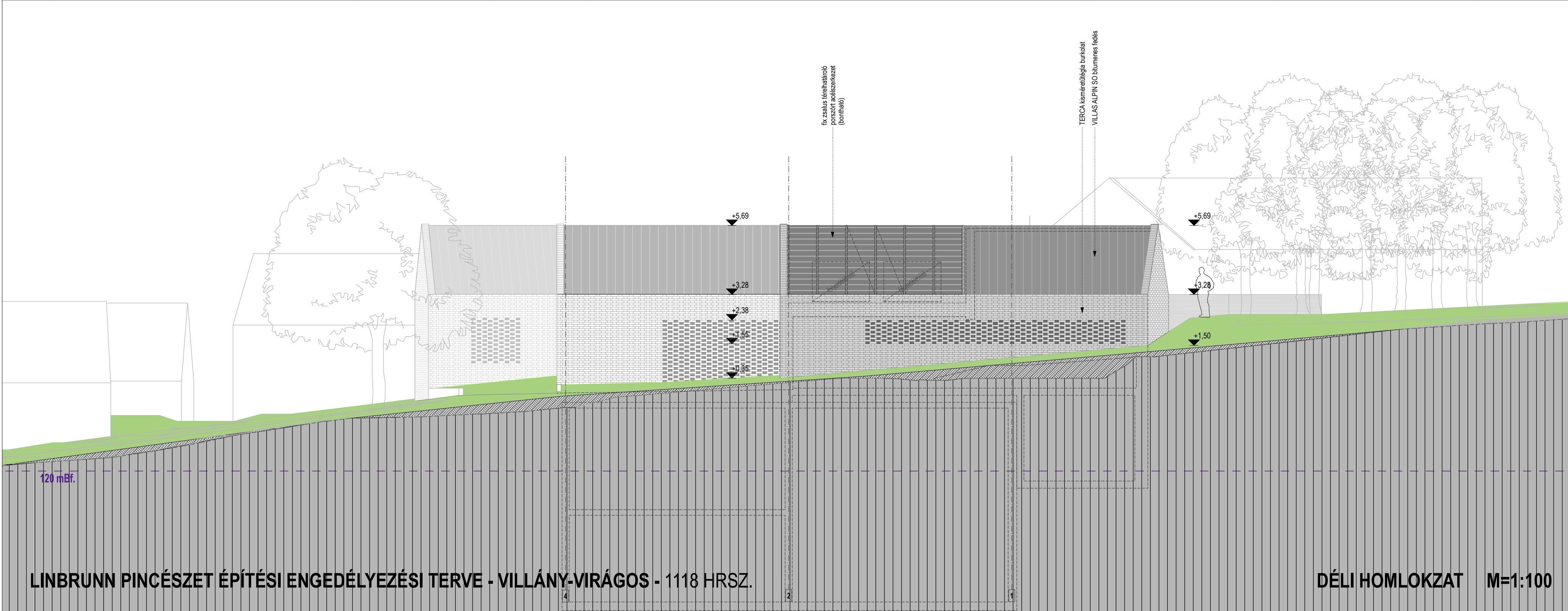
RAKTÁR ÉPÜLET ÉSZAKI HOMLOKZATA M=1:100
