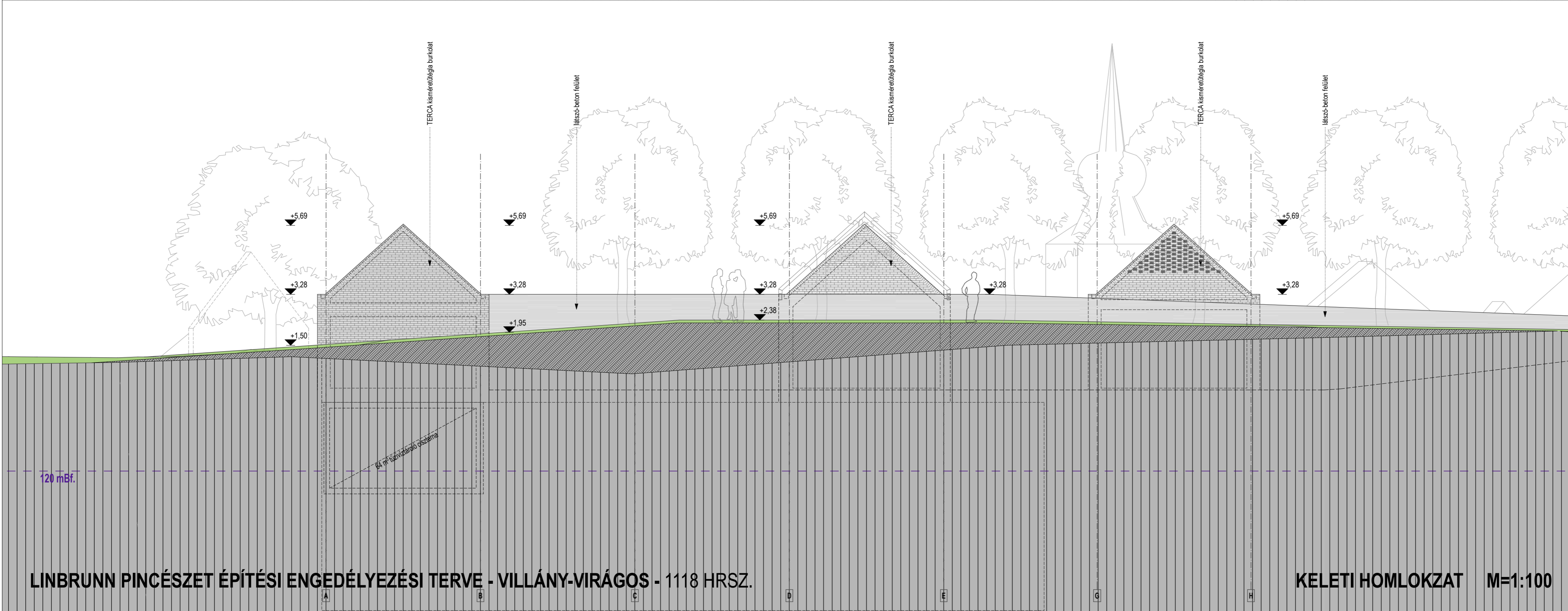
NYUGATI HOMLOKZAT M=1:100
