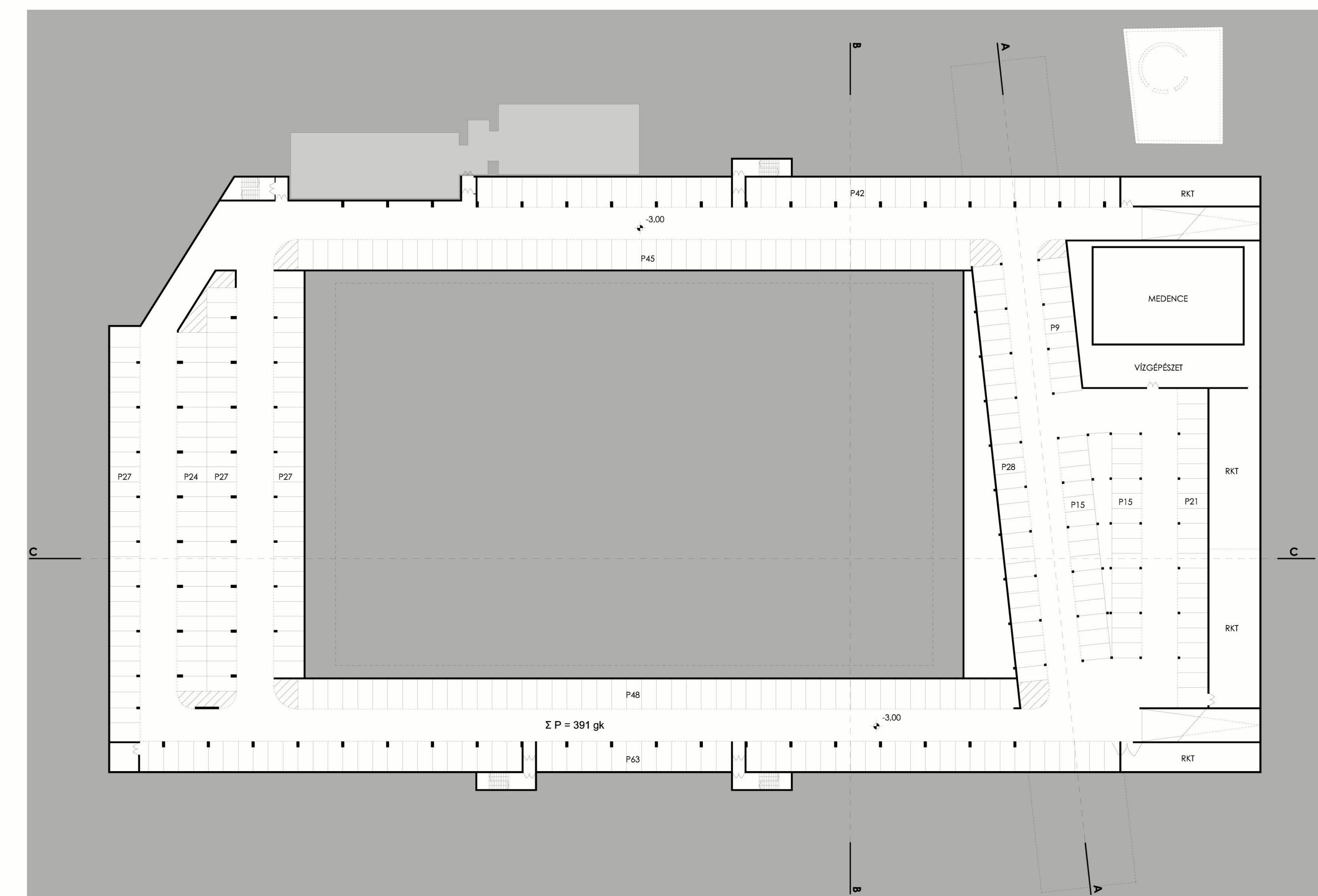
PARKOLÓSZINTI ALAPRAJZ
