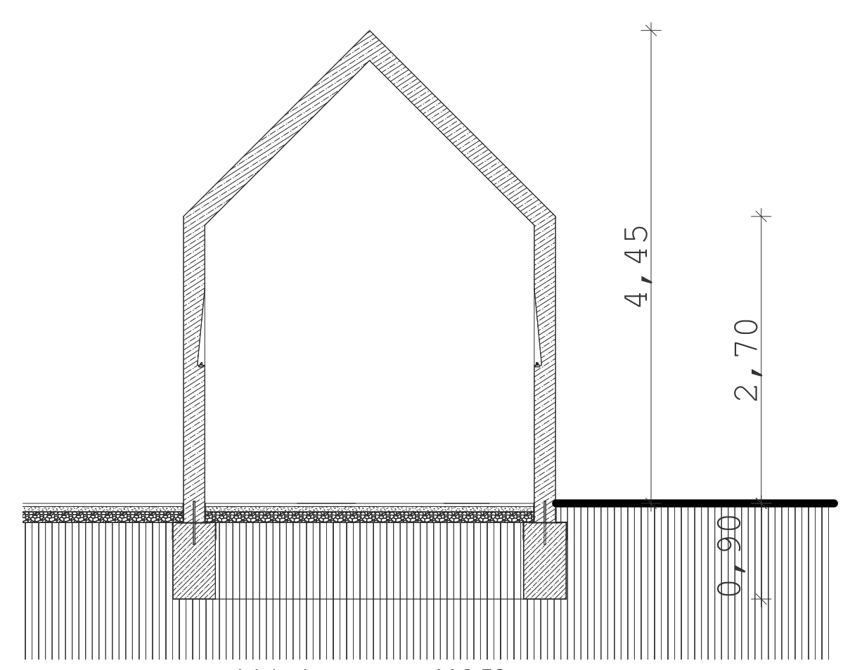
A kápolna metszete M 1:50
