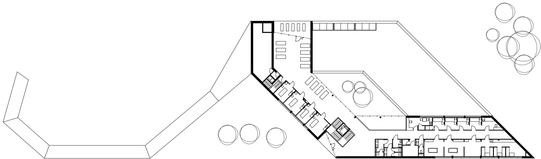
Pápa, Gyógy- és termálfürdő, Gyógyászat emeleti alaprajz
