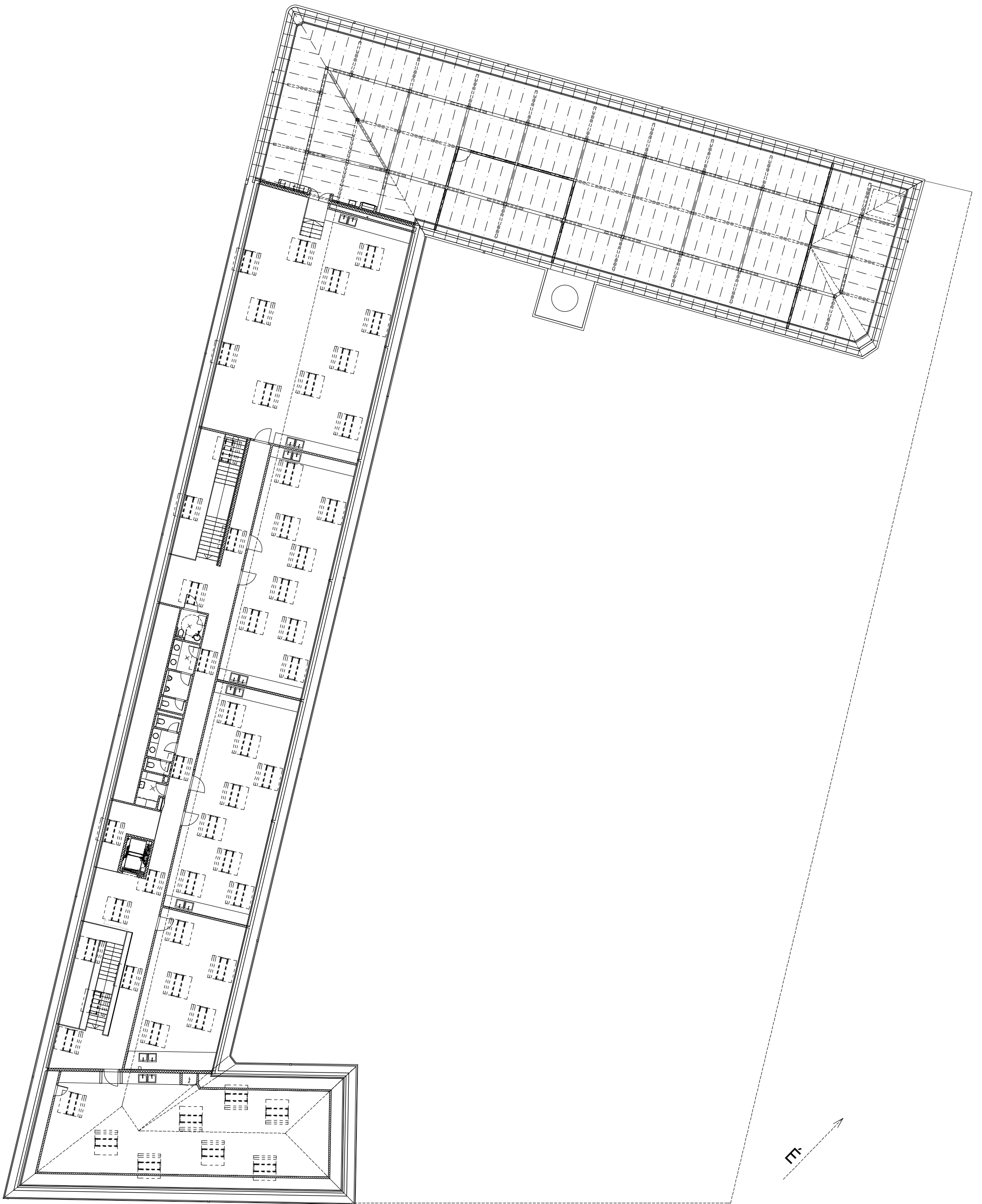
+2. SZINT - FESTŐ MŰTERMEK, GÉPÉSZET
