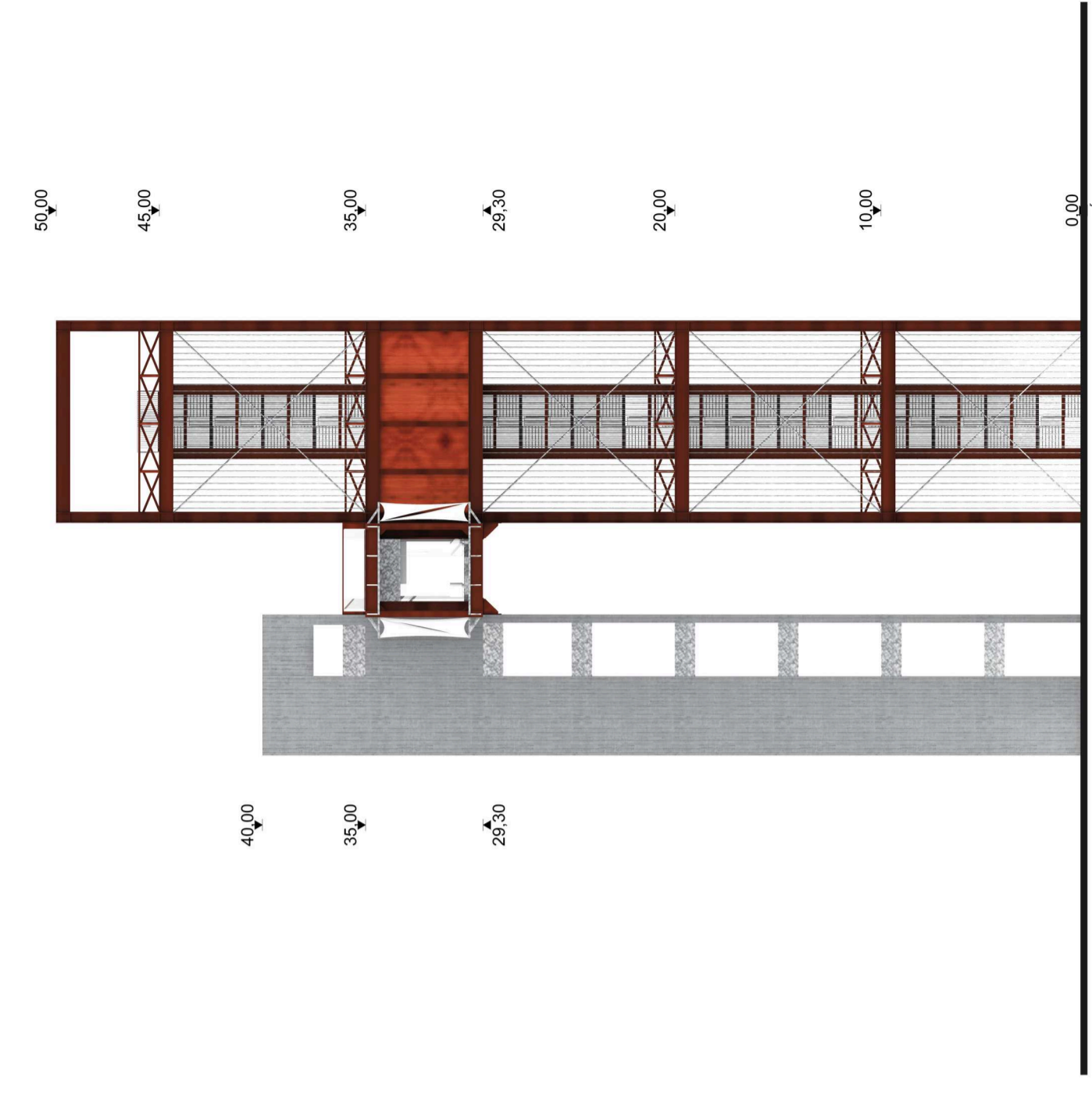
Nyugati homlokzat
