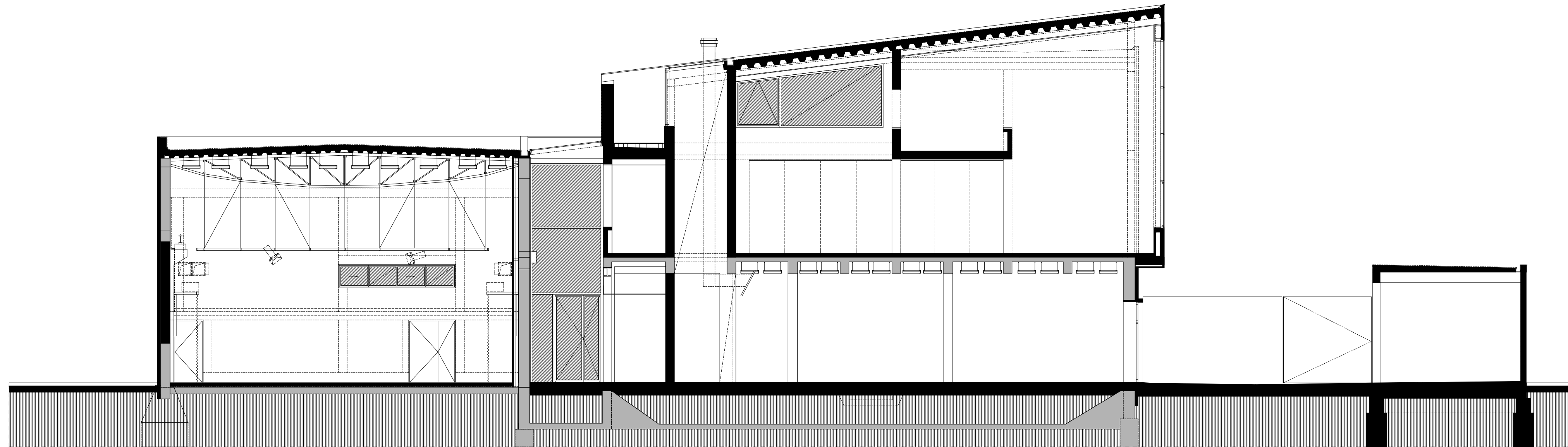
A-A METSZET
