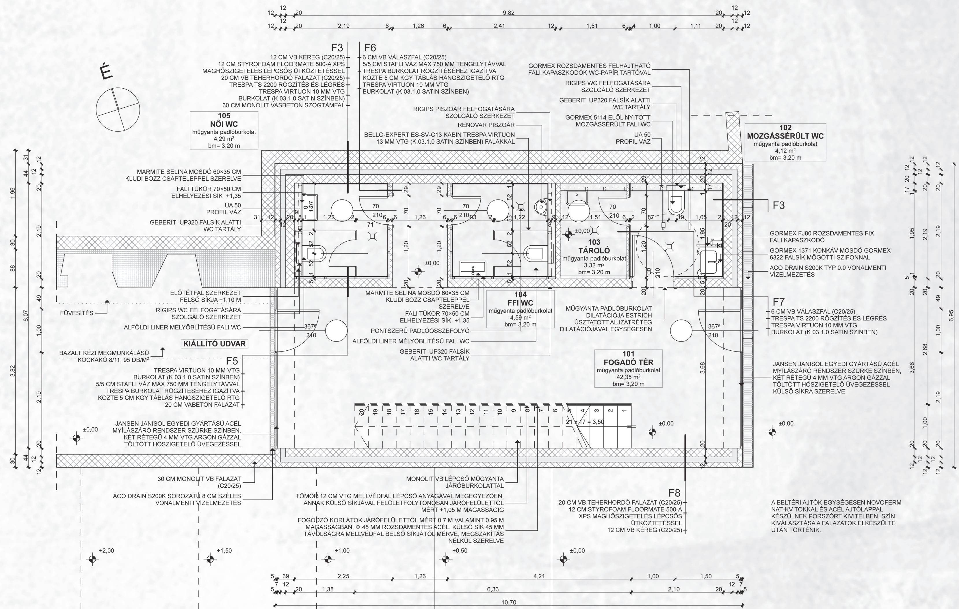
Földszinti alaprajzi részlet | M=1:50
