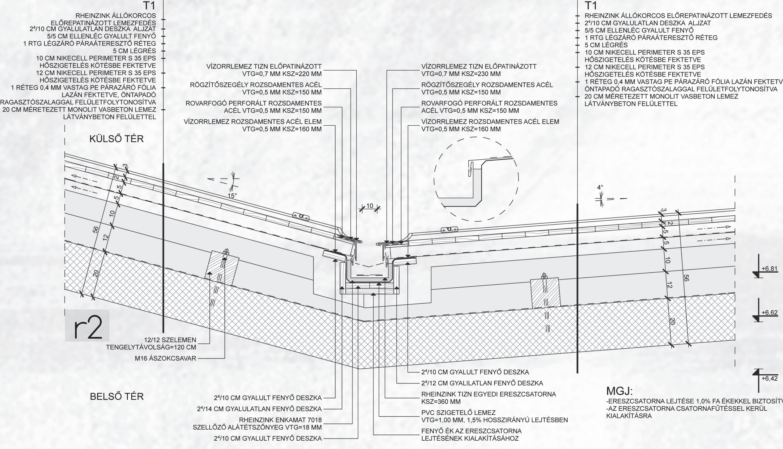
Részletrajzok | M=1:10
