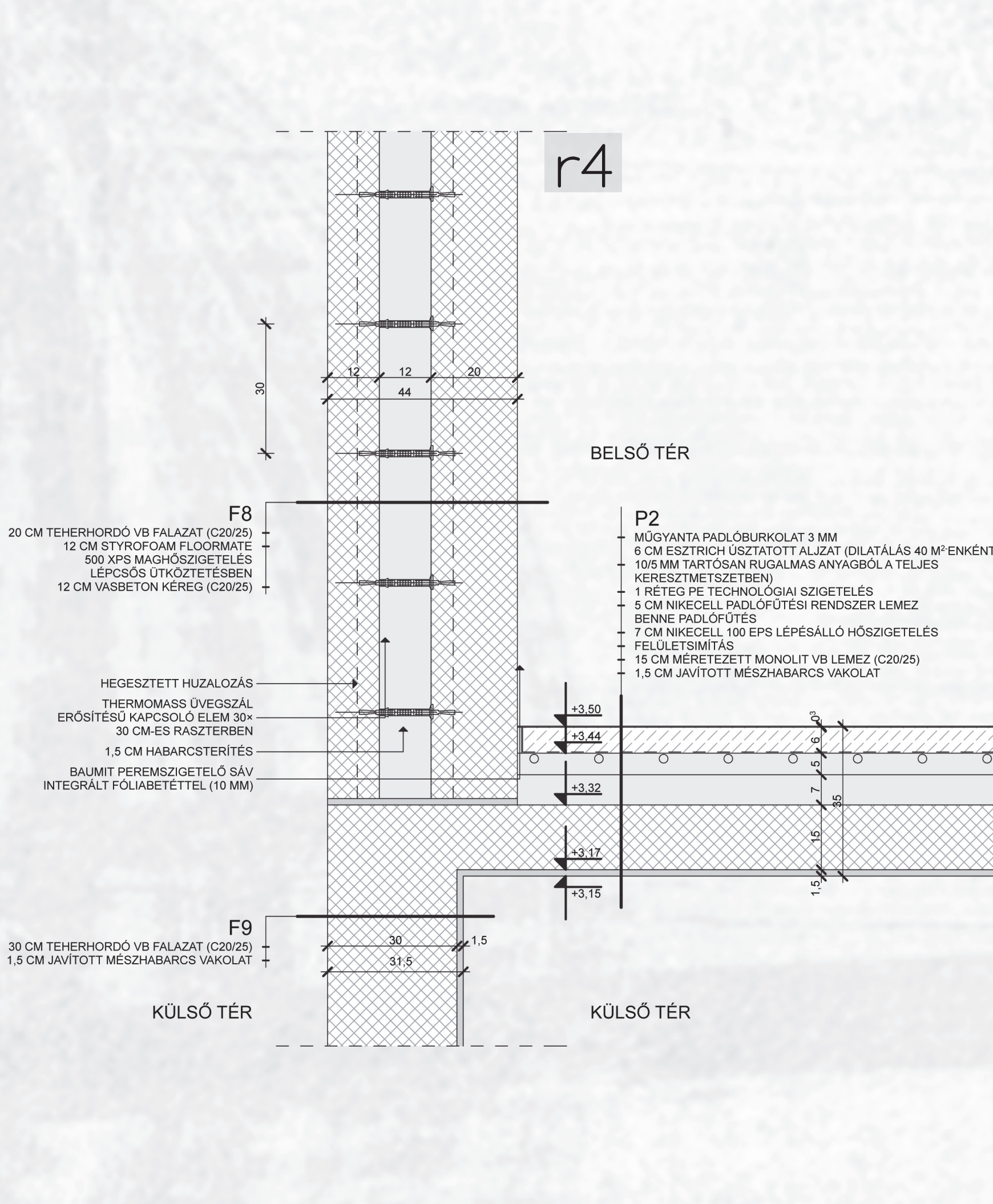
Részletrajzok | M=1:10
