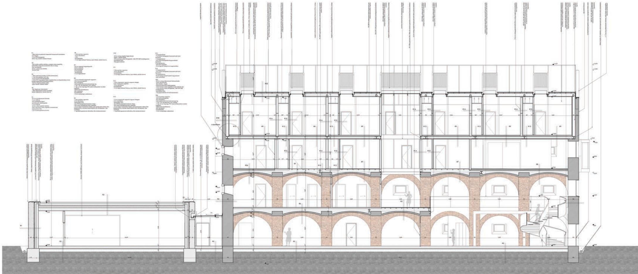
B-B metszet
