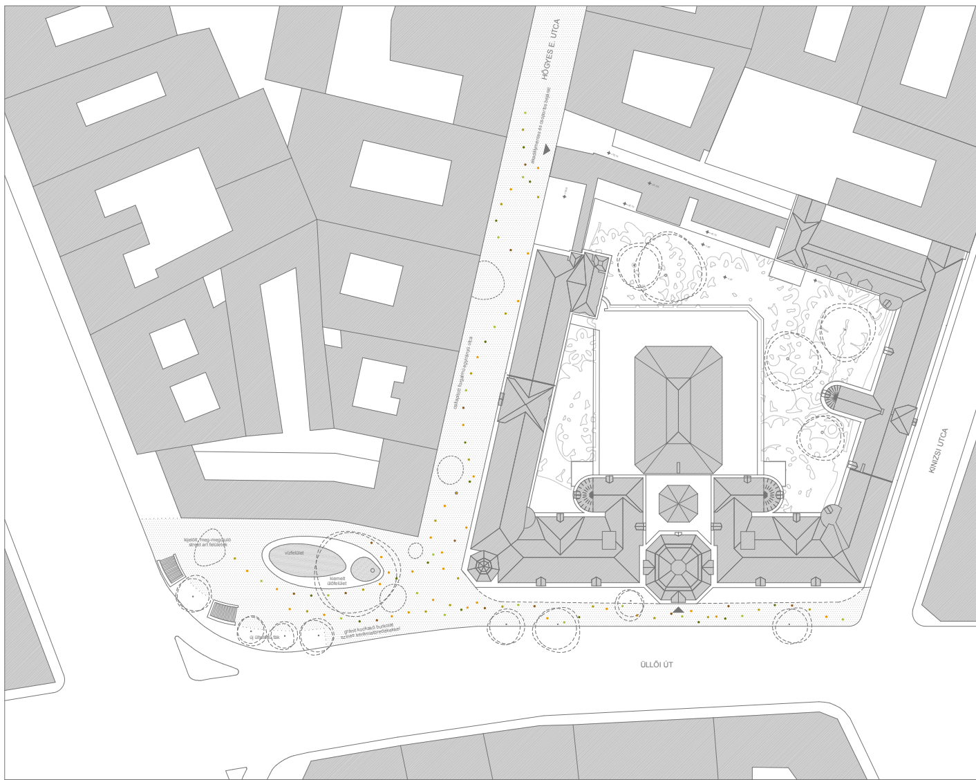
HELYSZÍNRAJZ 1:500
