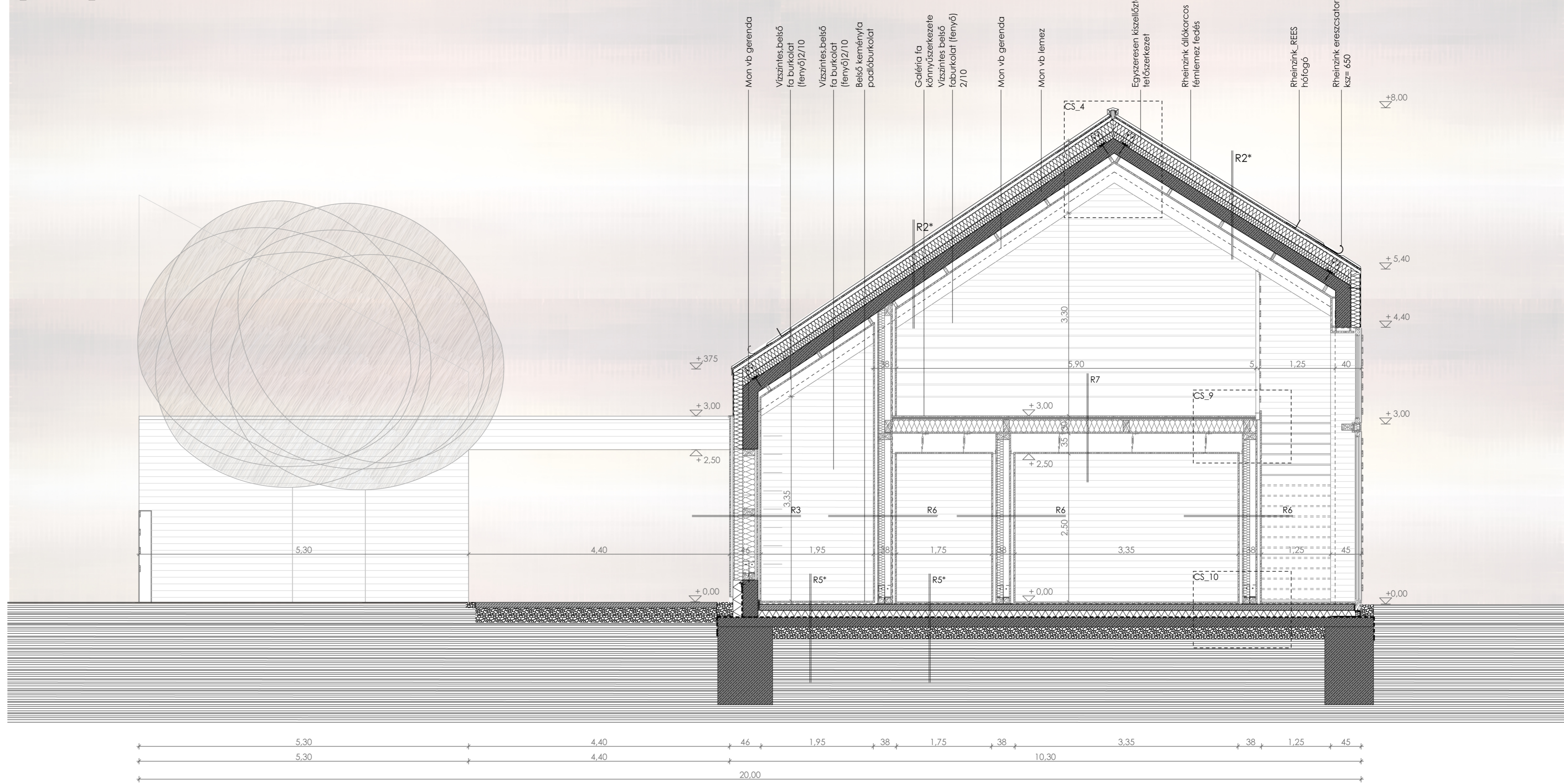
C_C metszet_M 1:50
