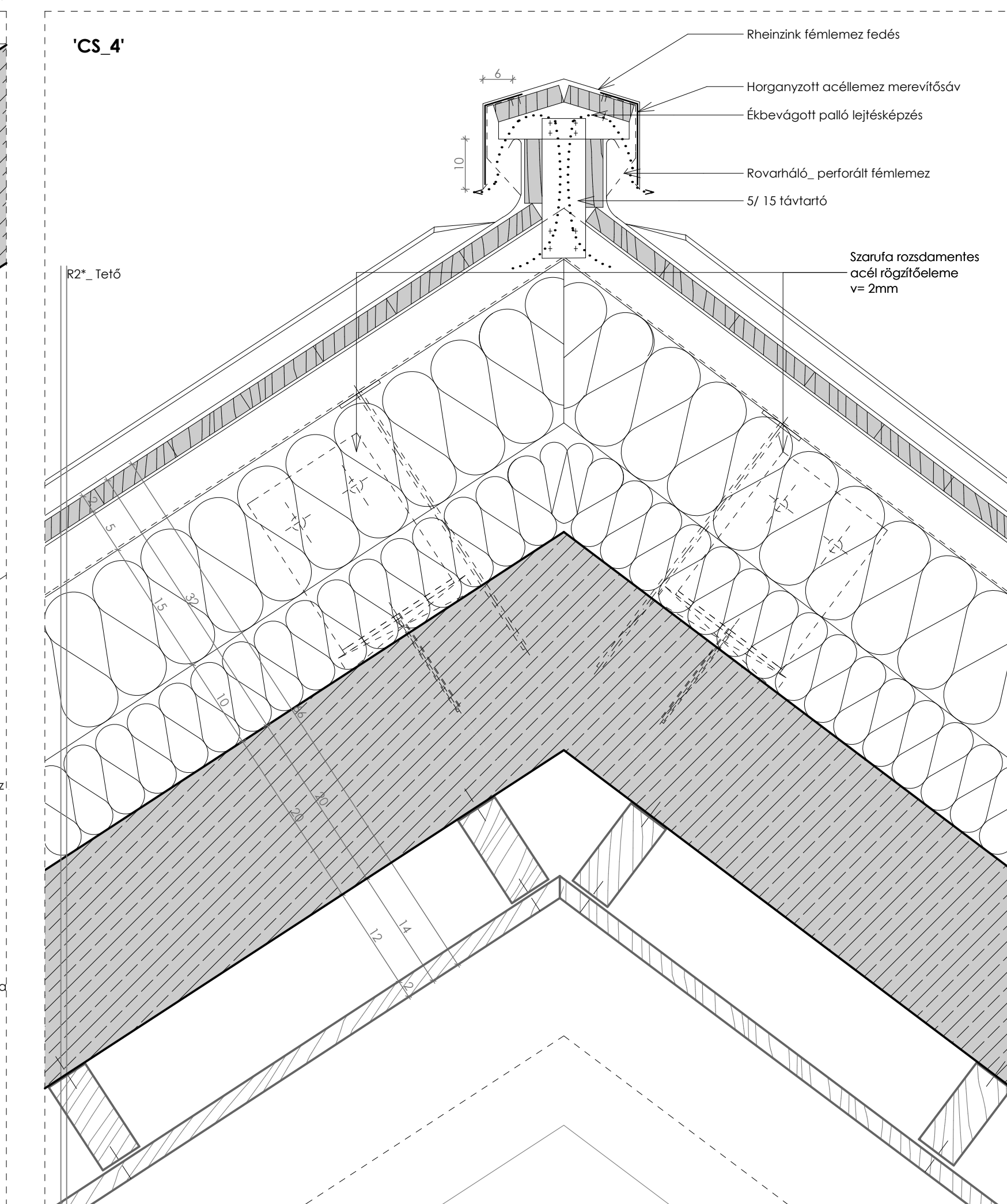
RÉSZLETRAJZOK_ M 1:5 ALAPÍTÁNYI FÓRUM_ GÖDÖLLŐ
