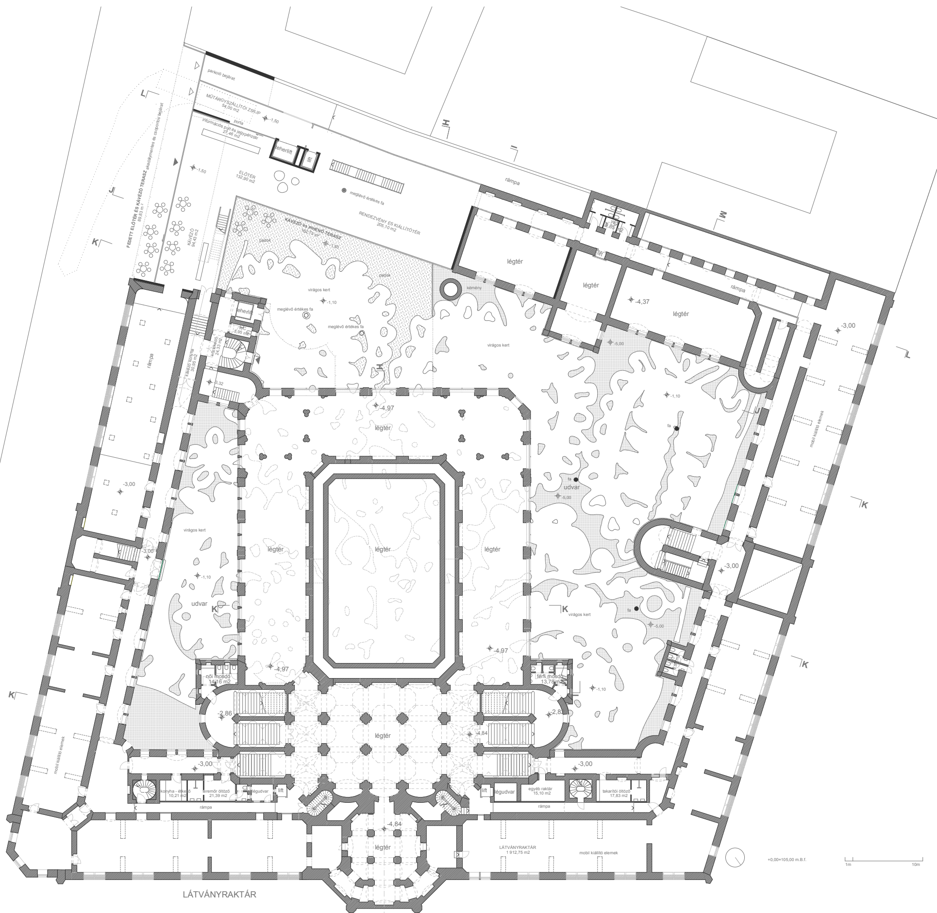
UTCASZINTI ALAPRAJZ 1:200
