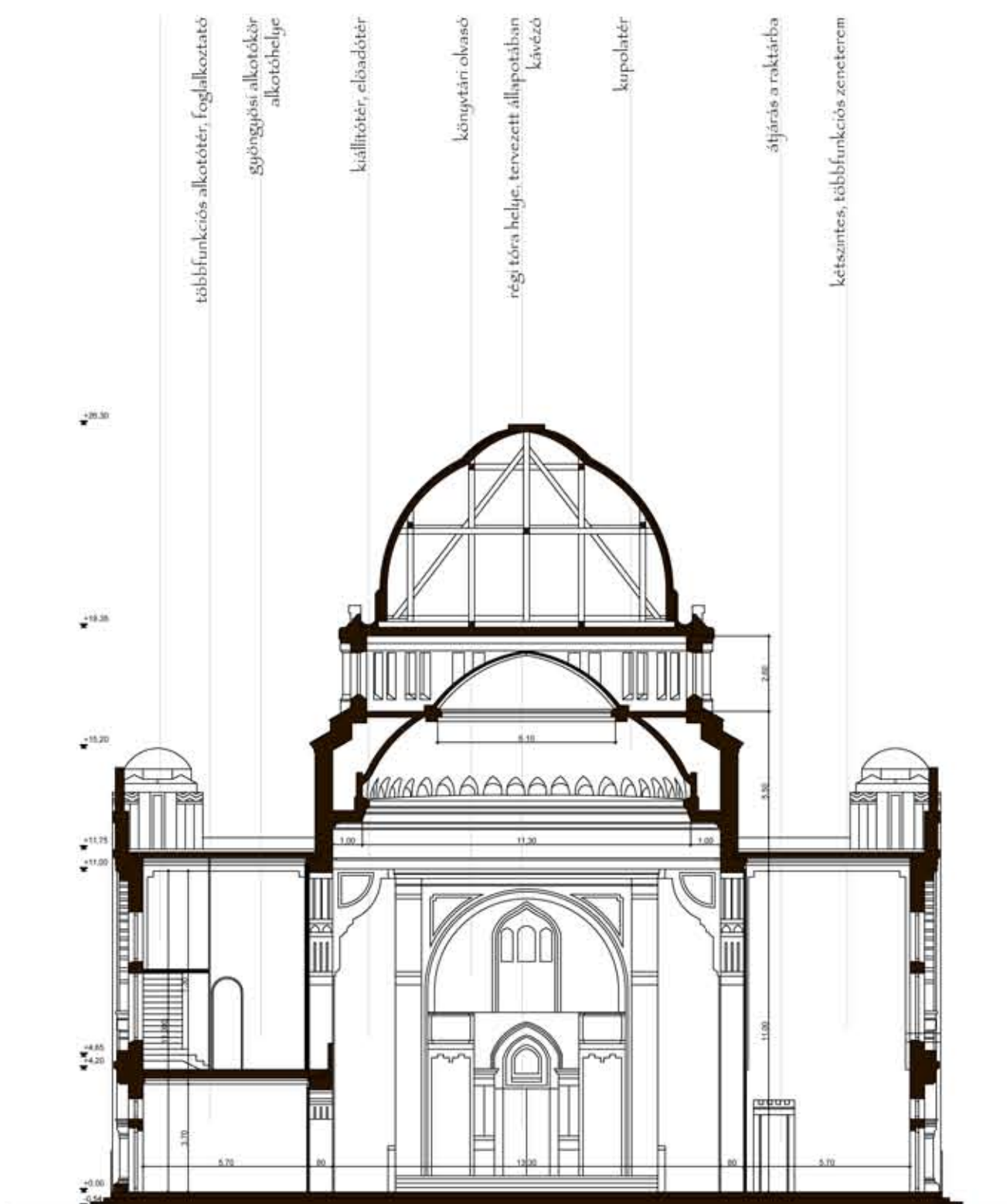
METSZET M1: 200
