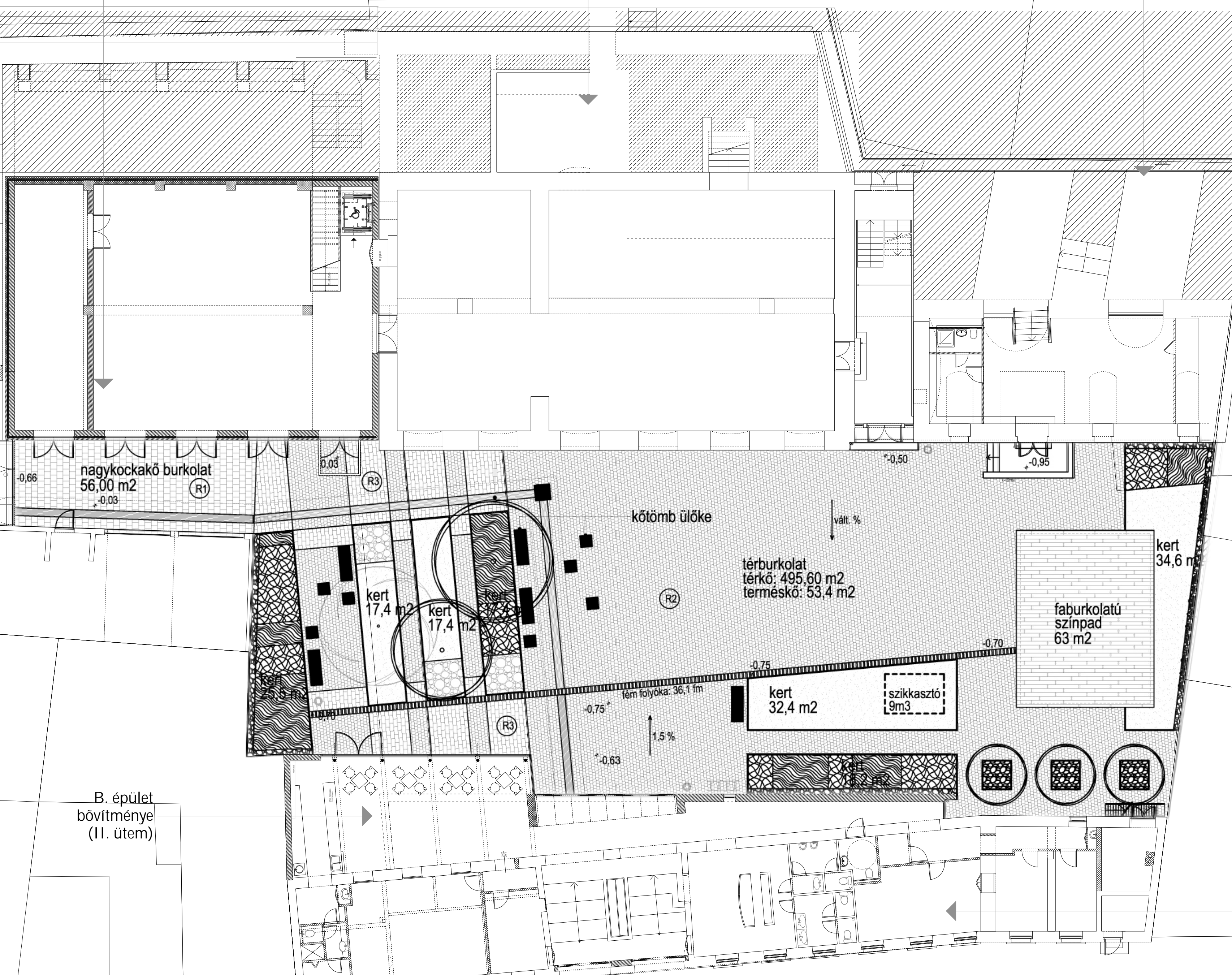
földszint átnézeti alaprajza
