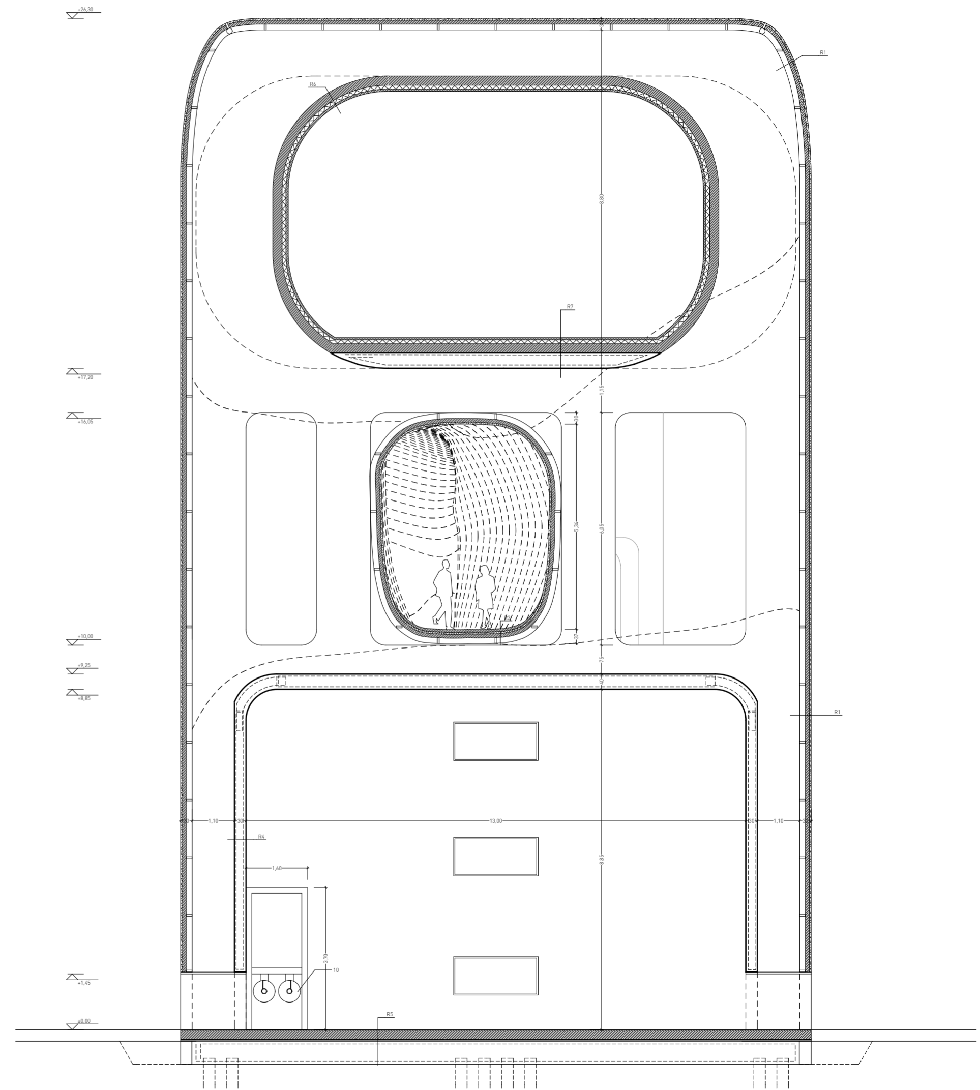
Keresztmetszet 6. / Tervlap 3.6
