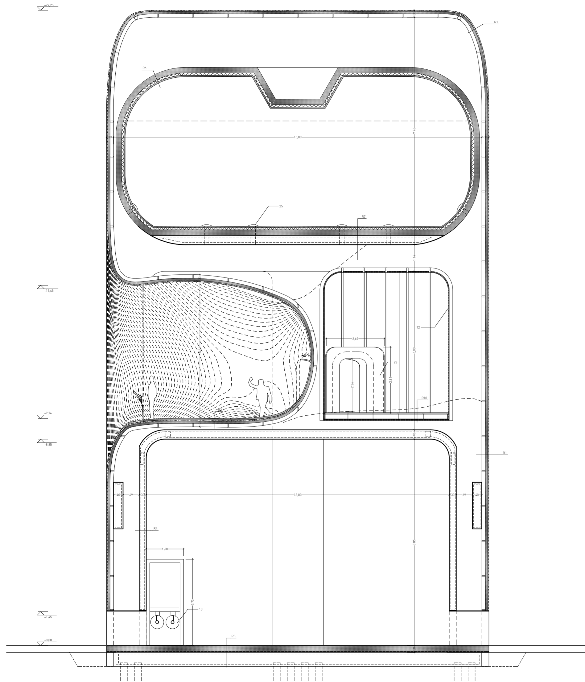
Keresztmetszet 5. / Tervlap 3.5
