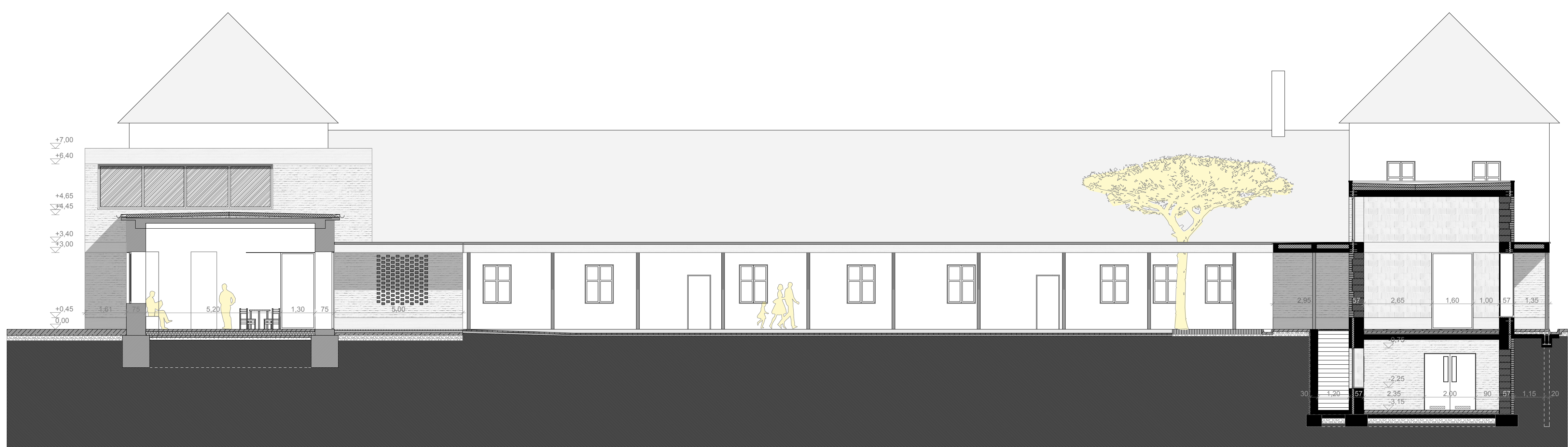
A/3 METSZET ÉS BELSŐ NYUGATI HOMLOKZAT
