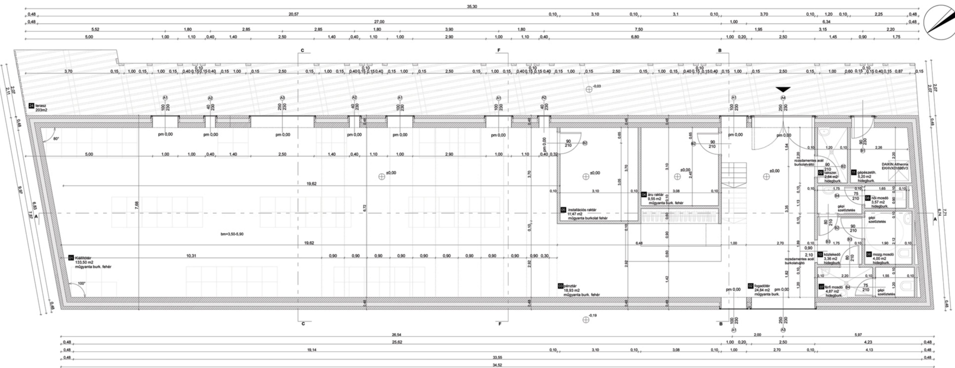
Alaprajz M=1:50
