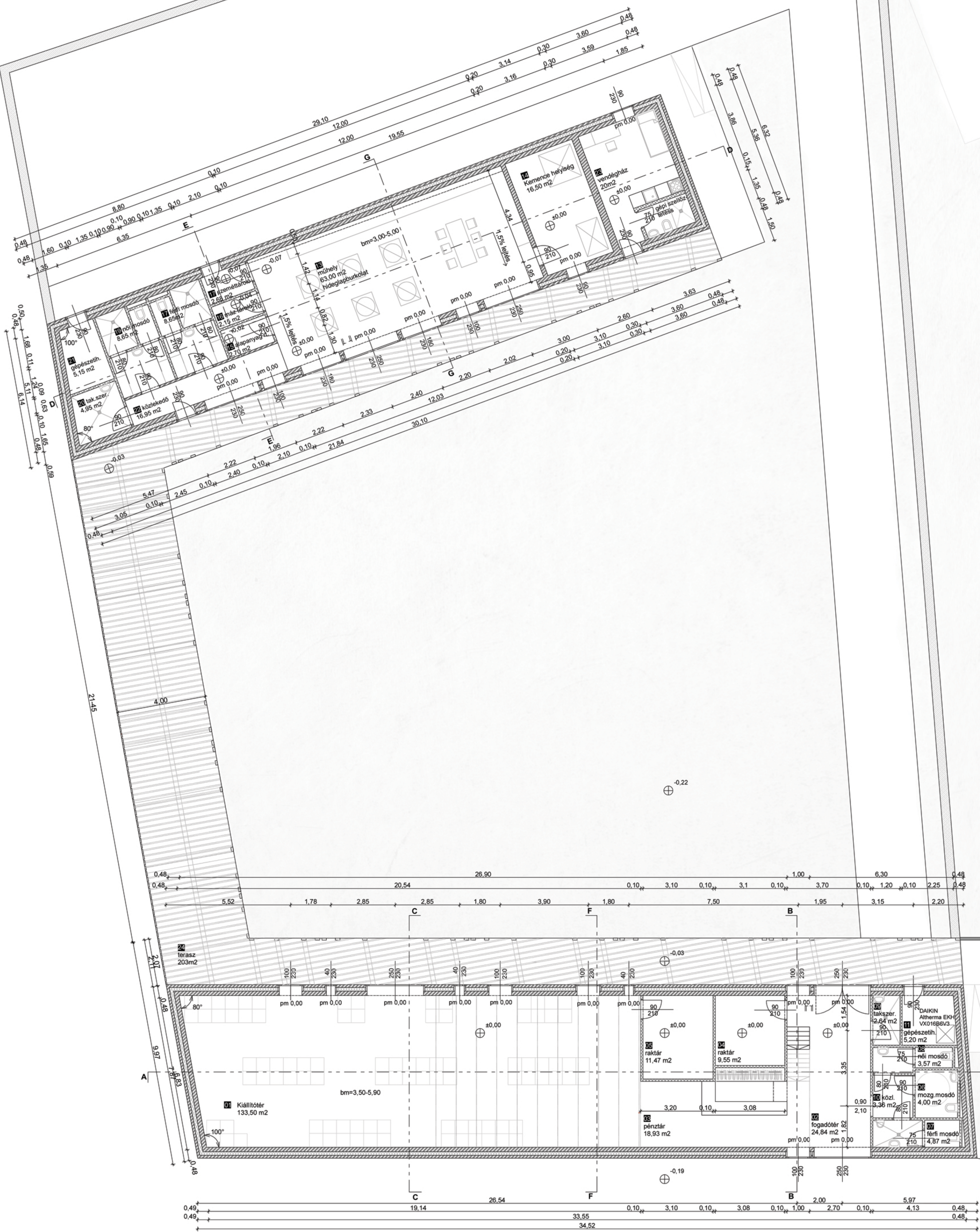
Alaprajz M=1:100
