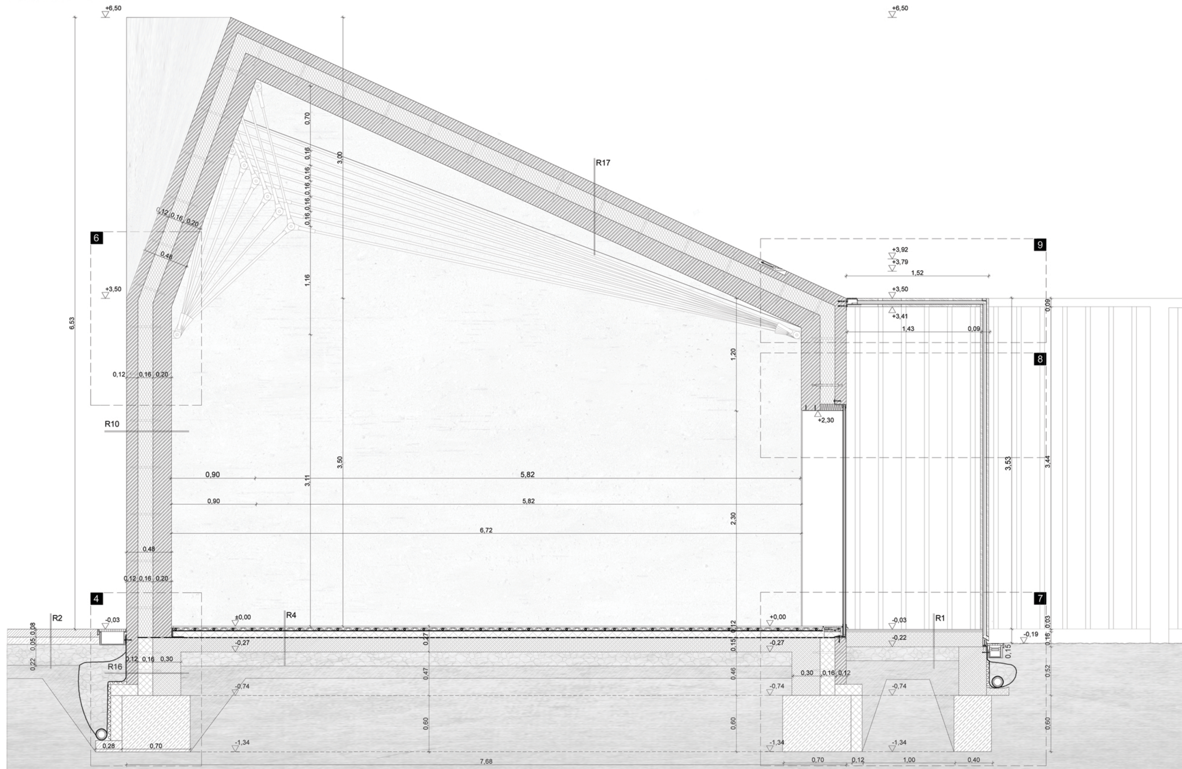
F-F metszet M=1:25
