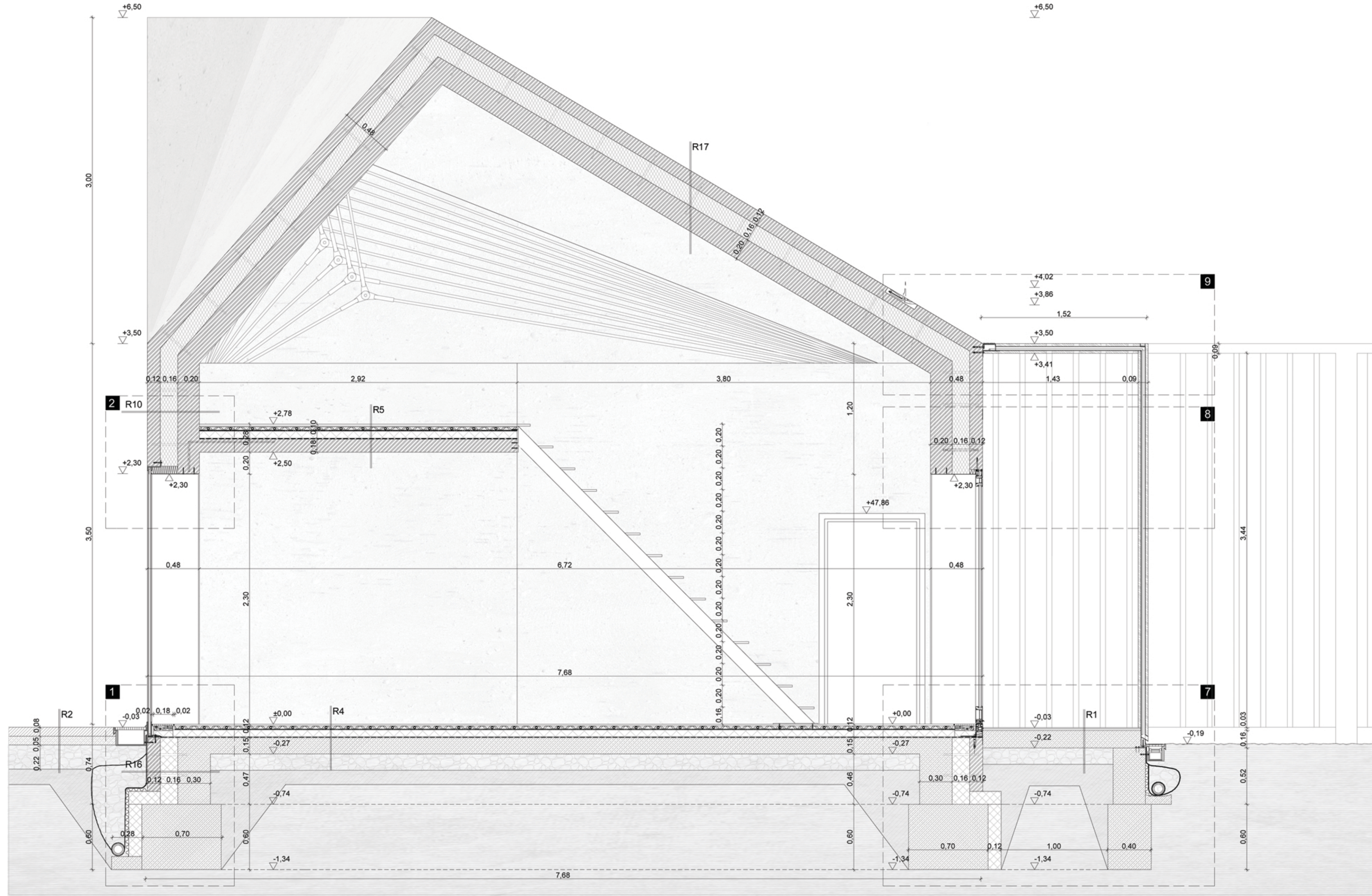
B-B metszet M=1:25
