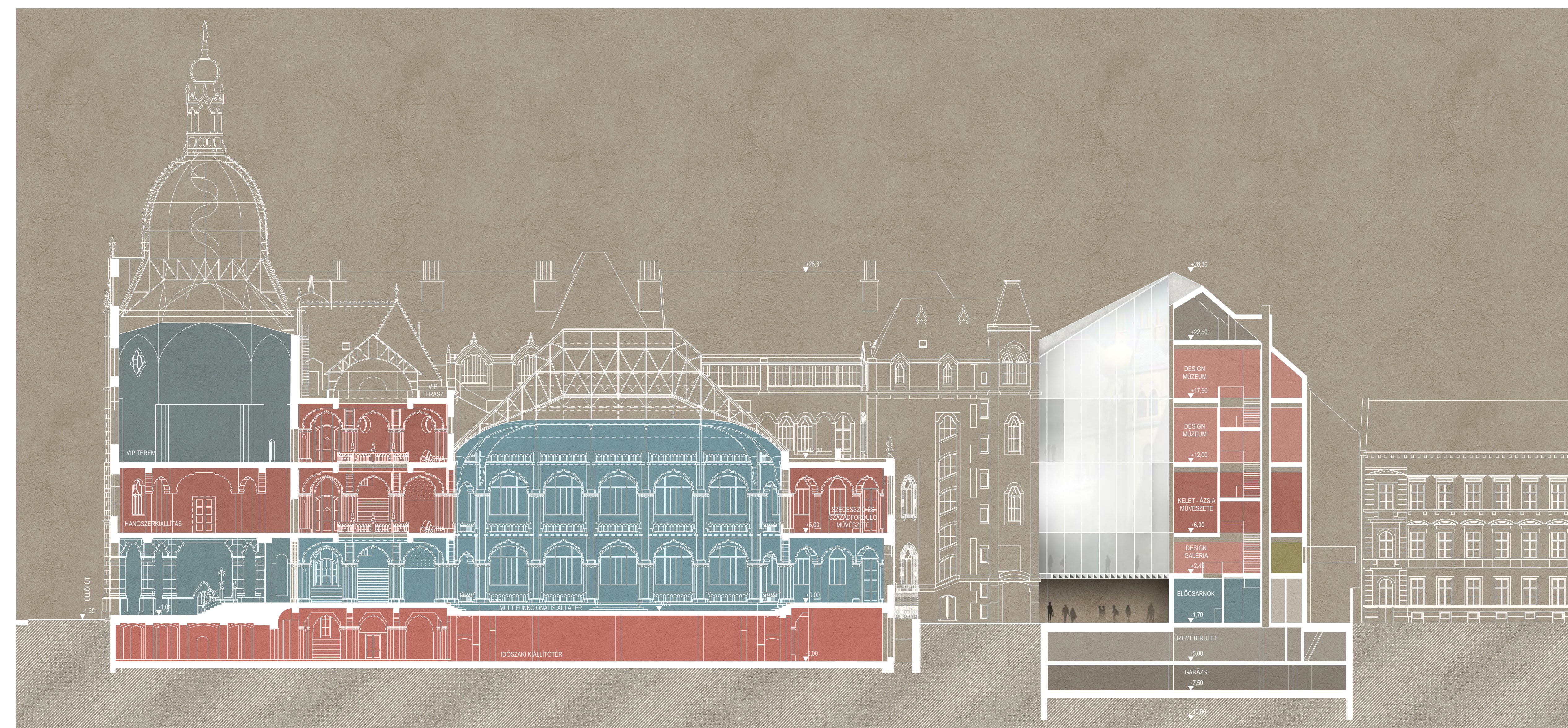
HOSSZMETSZET M=1:200
