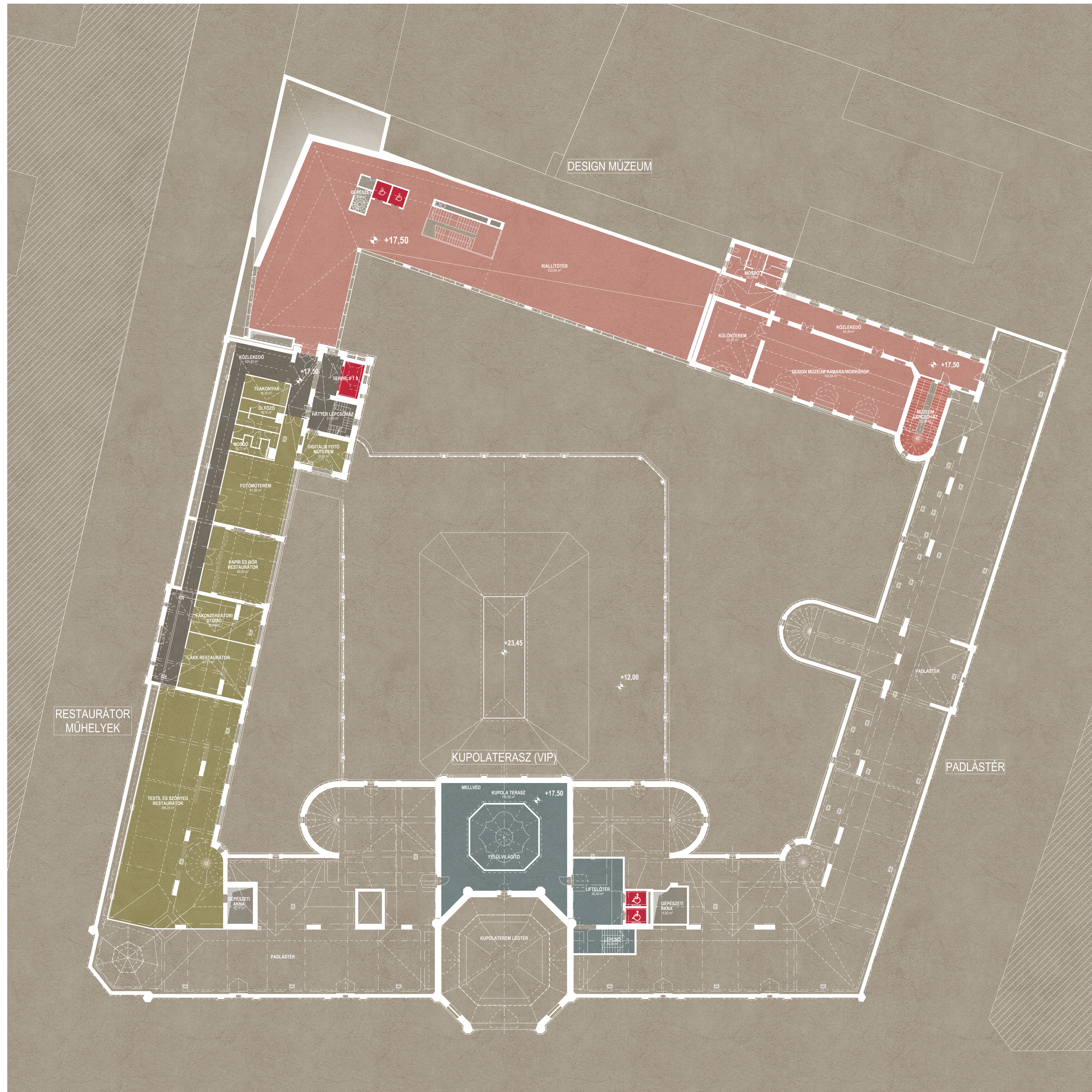
III. EMELETI ALAPRAJZ M=1:200
