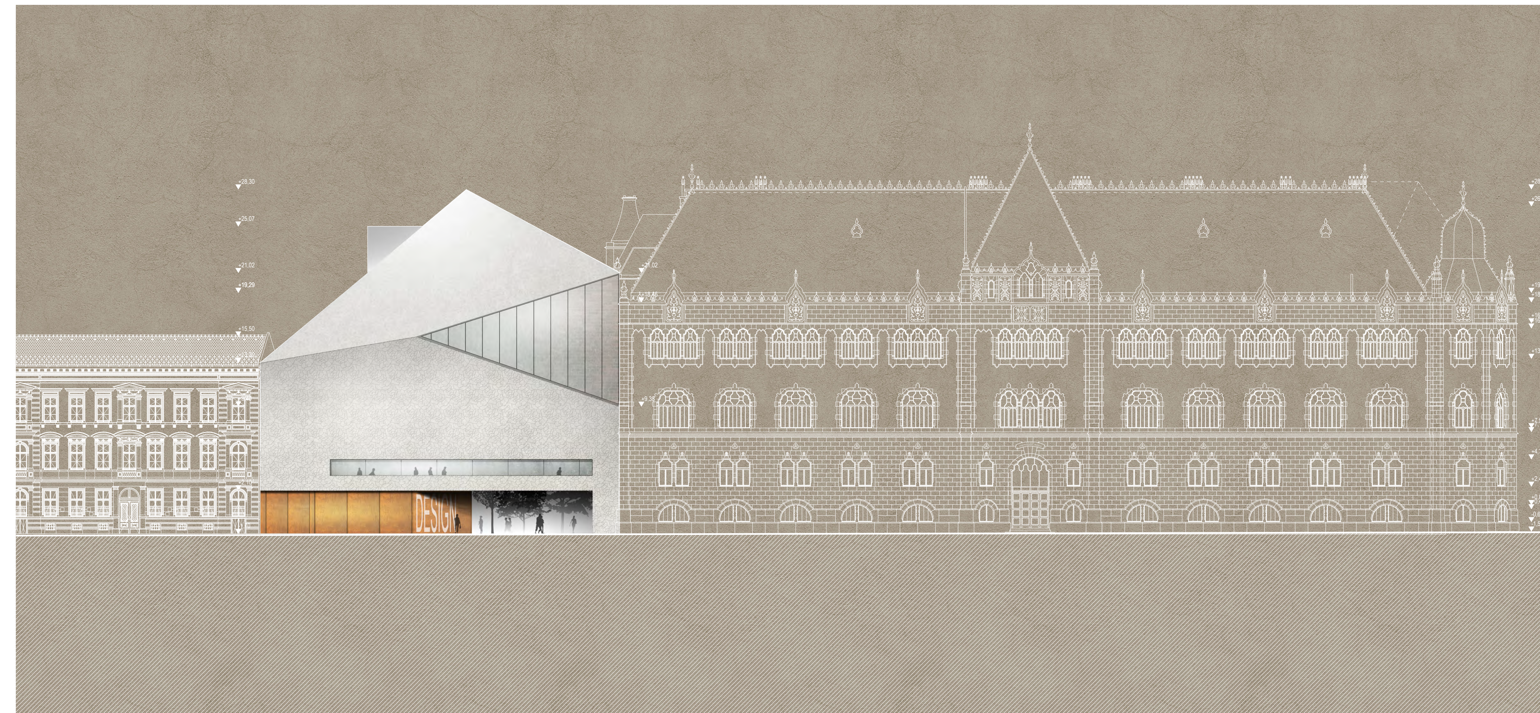
HÖGYES ENDRE UTCAI HOMLOKZAT M=1:200
