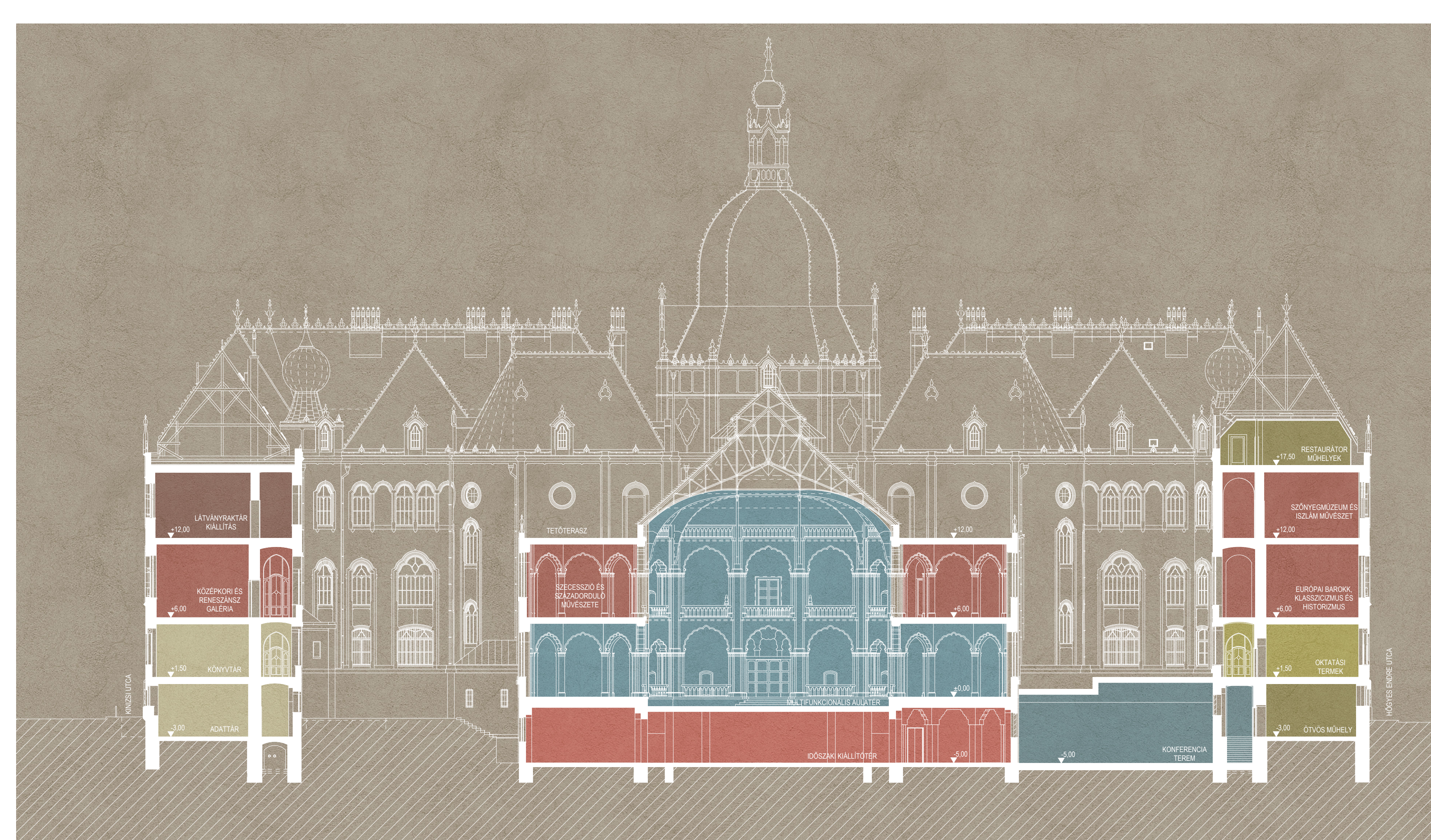
KERESZTMETSZET M=1:200
