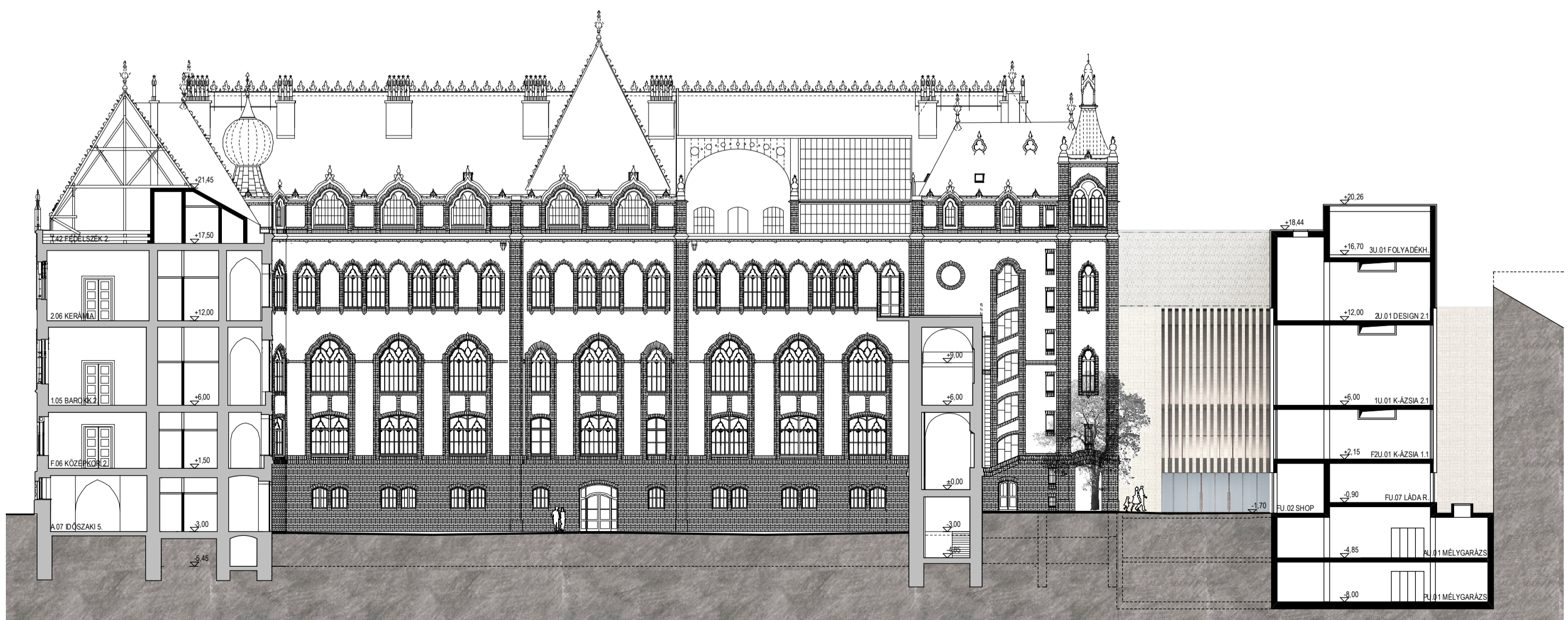
BELSŐ UDVARI HOMLOKZAT - HŐGYES UTCA M 1:200
