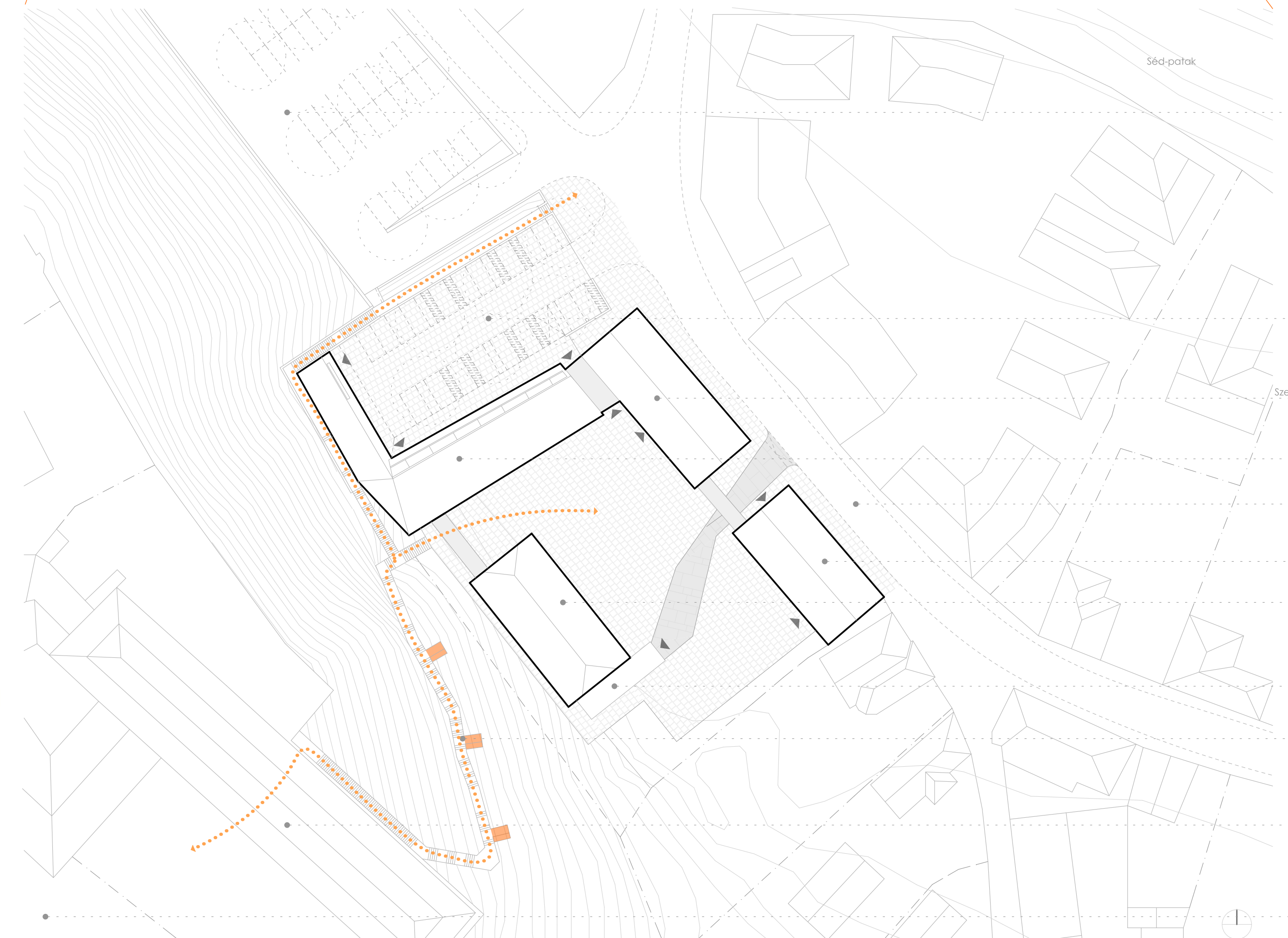
Helyszínrajz M 1:500
