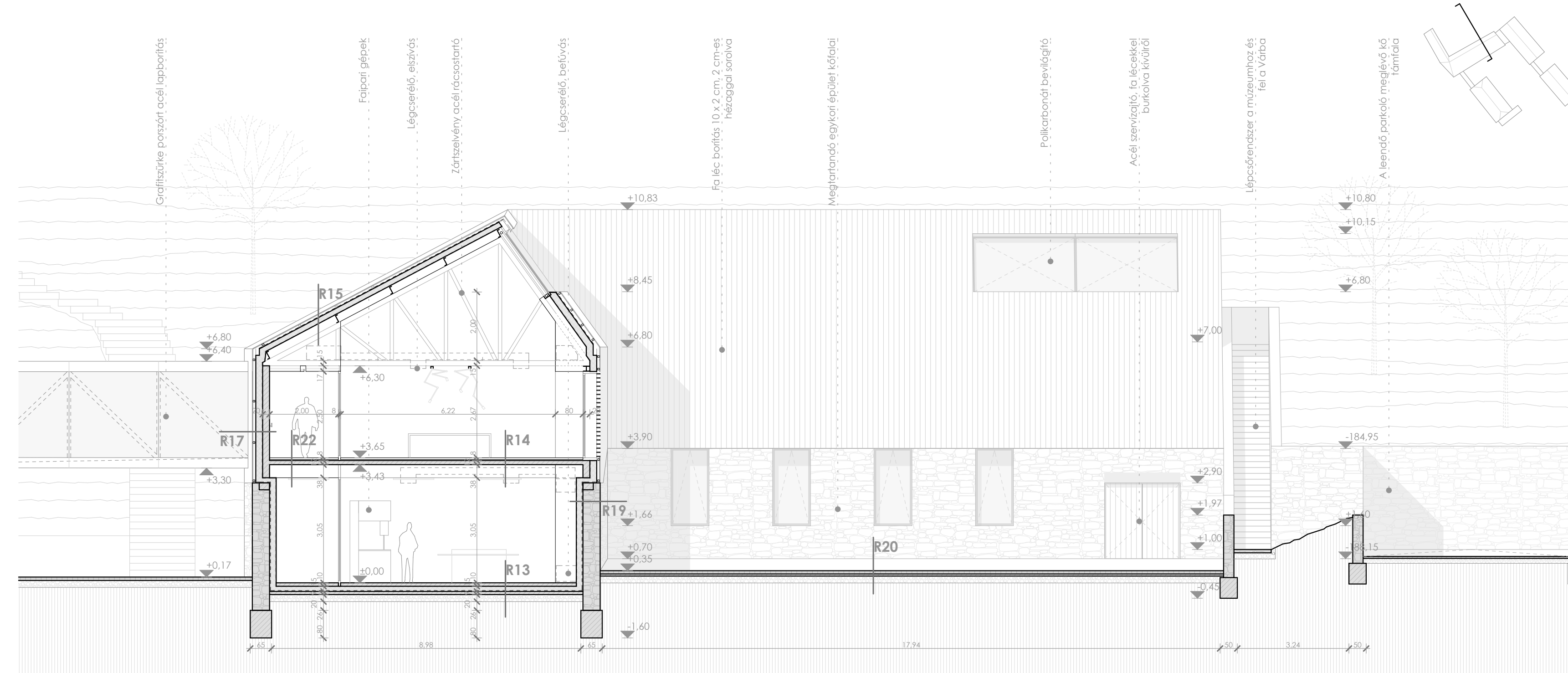
I-I metszet M 1:100
