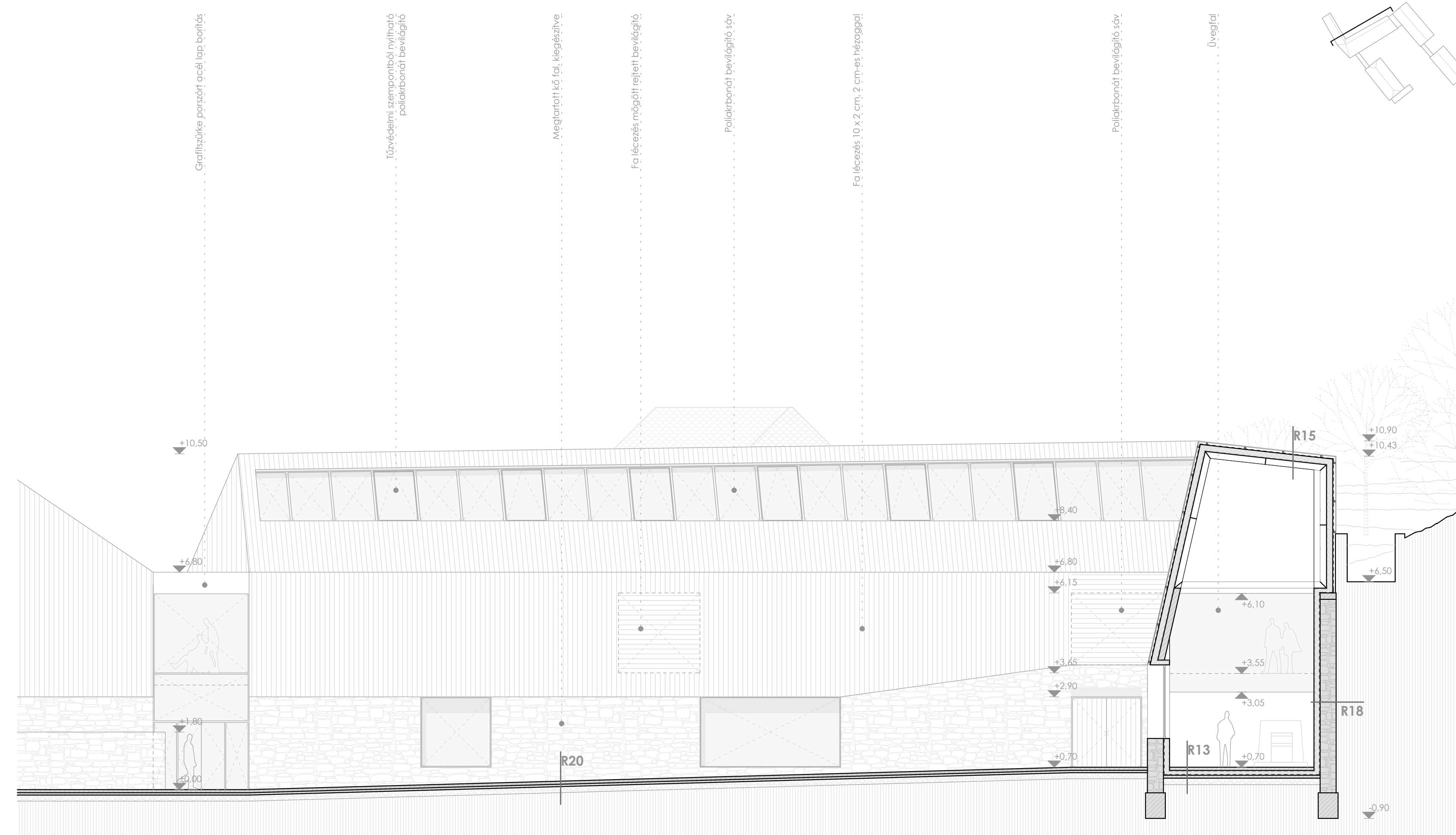
J-J metszet M 1:100
