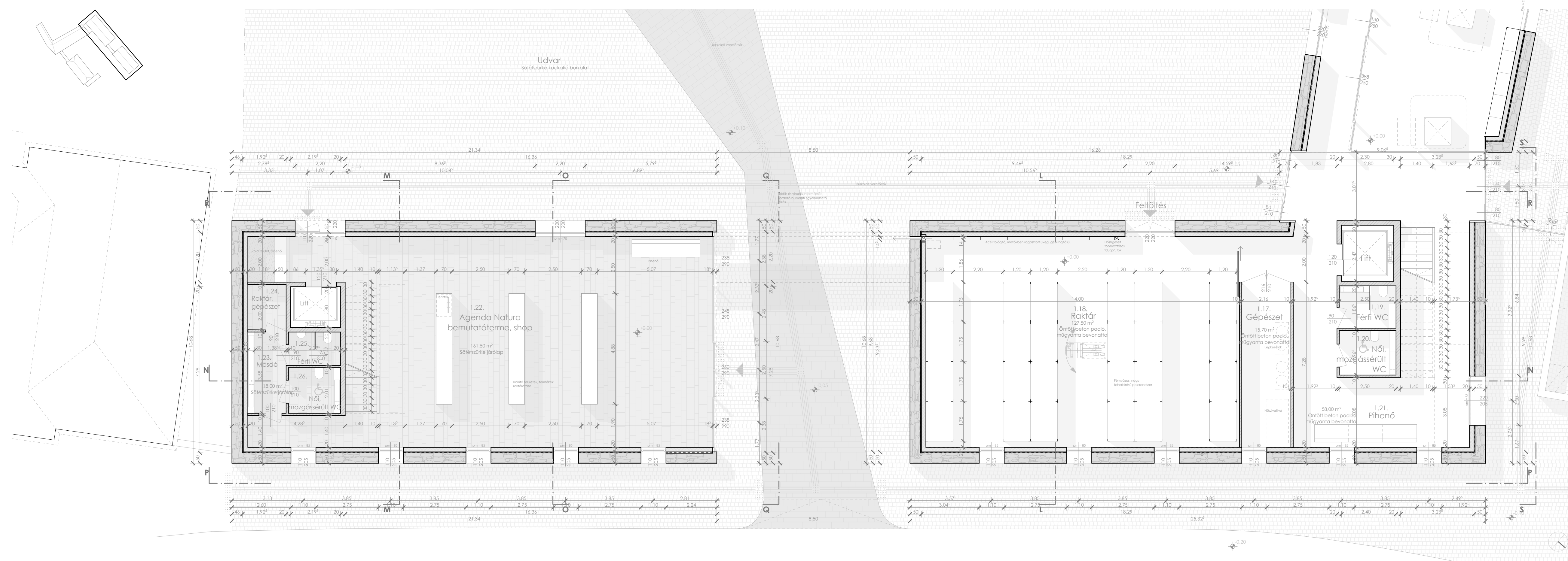
Földszinti alaprajzi részlet M 1:100
