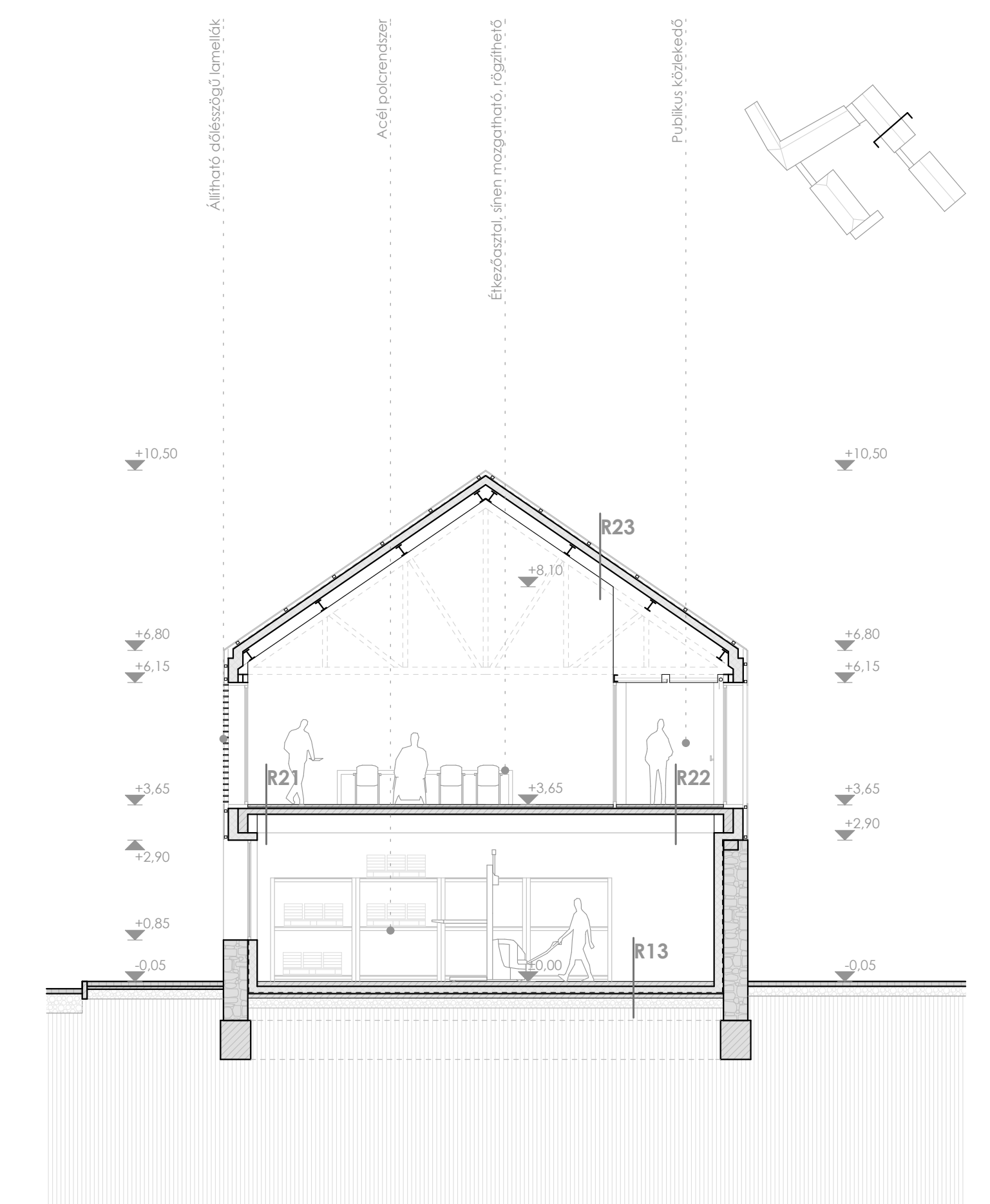
L-L metszet M 1:100
