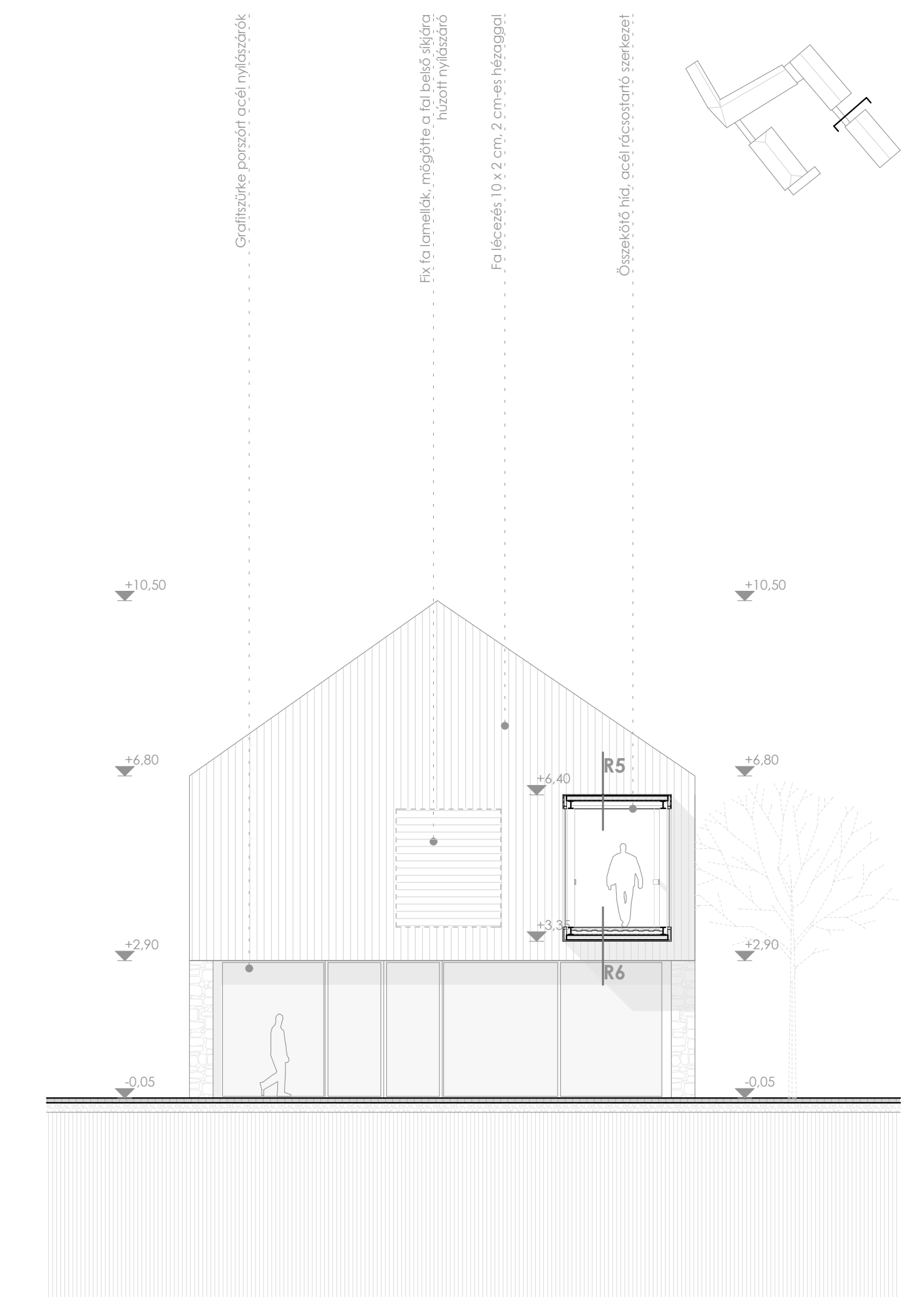
Q-Q metszet M 1:100
