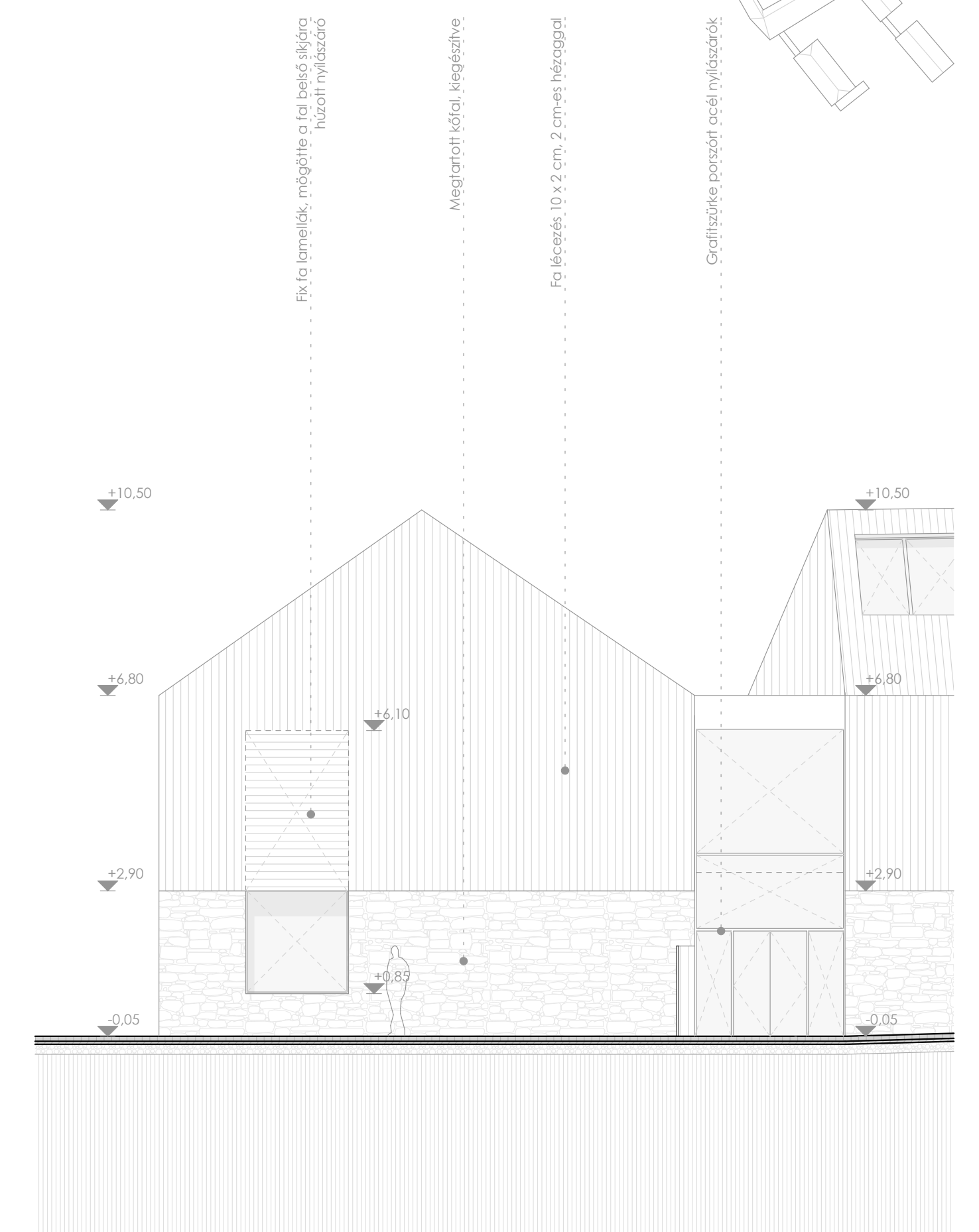
S-S metszet M 1:100
