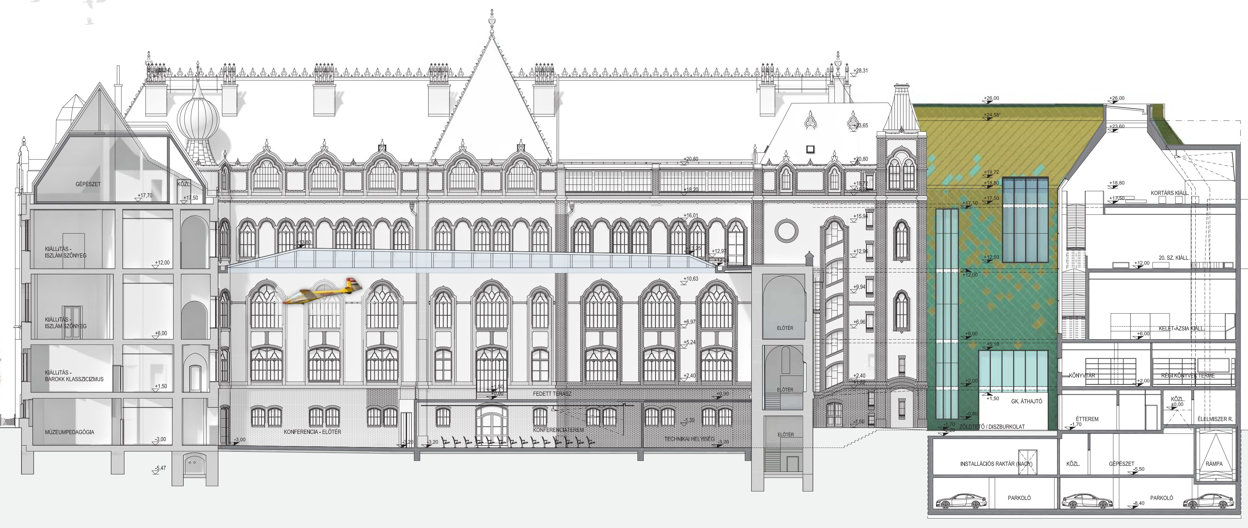
METSZET 4. 1=200
