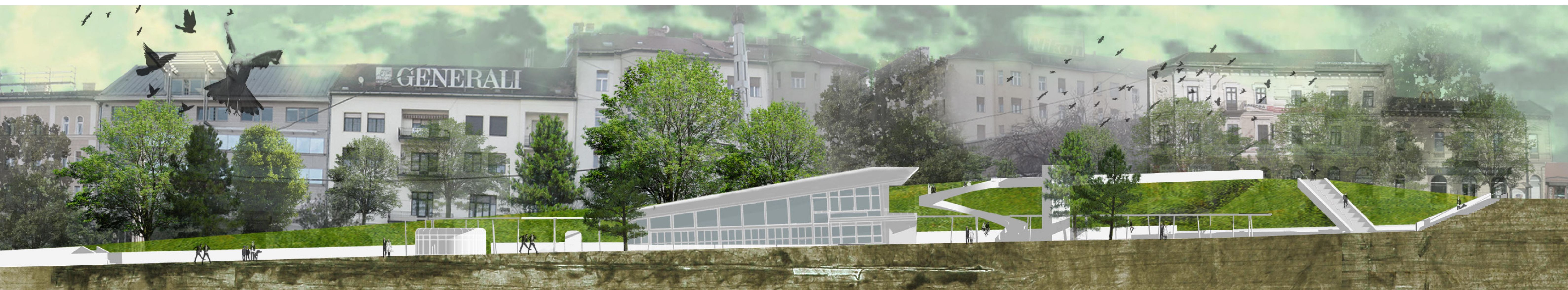
3.3. B-B TÉRMETSZET M 1:200
