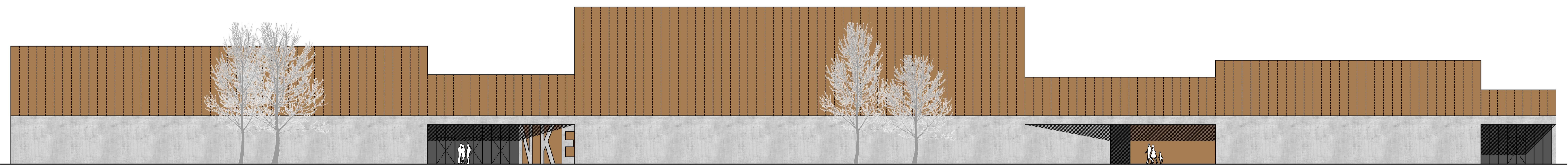
DIÓSZEGHY SÁMUEL UTCAI HOMLOKZAT m 1:200
