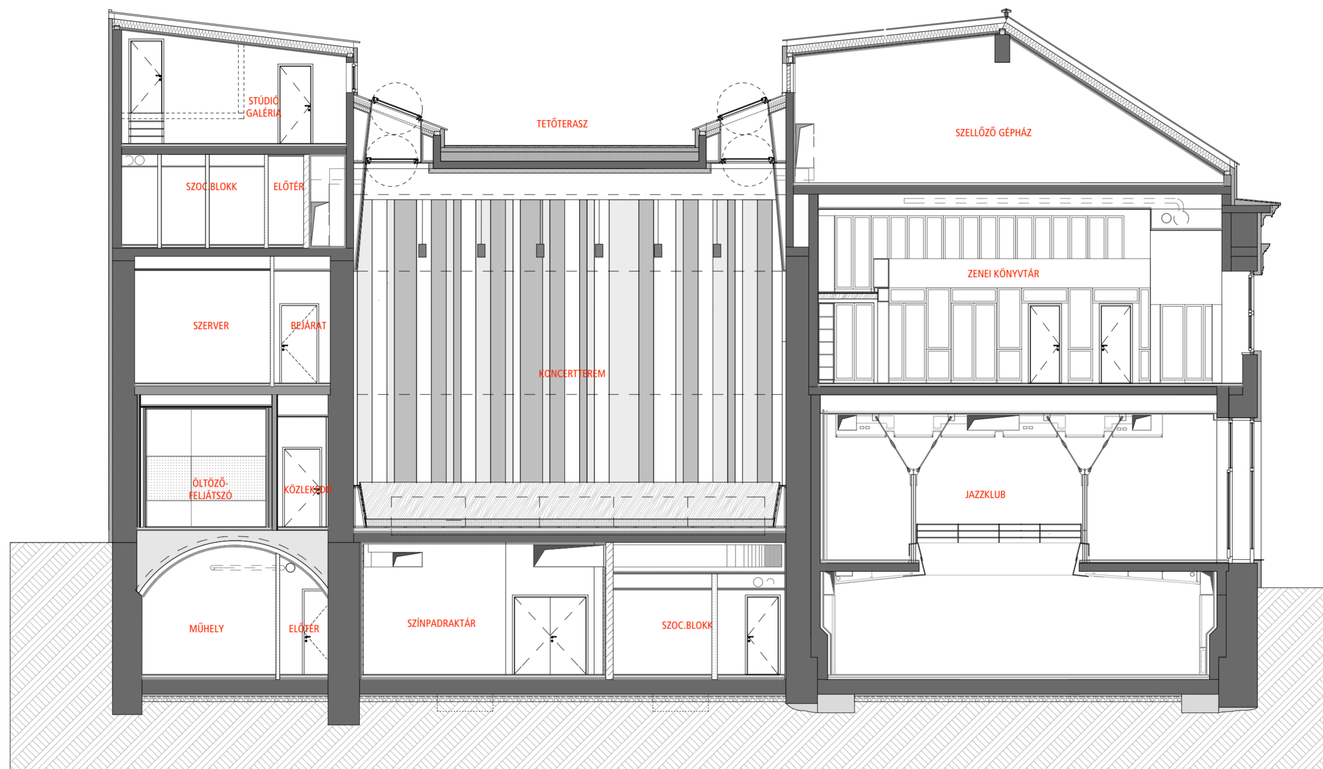
A-A METSZET
