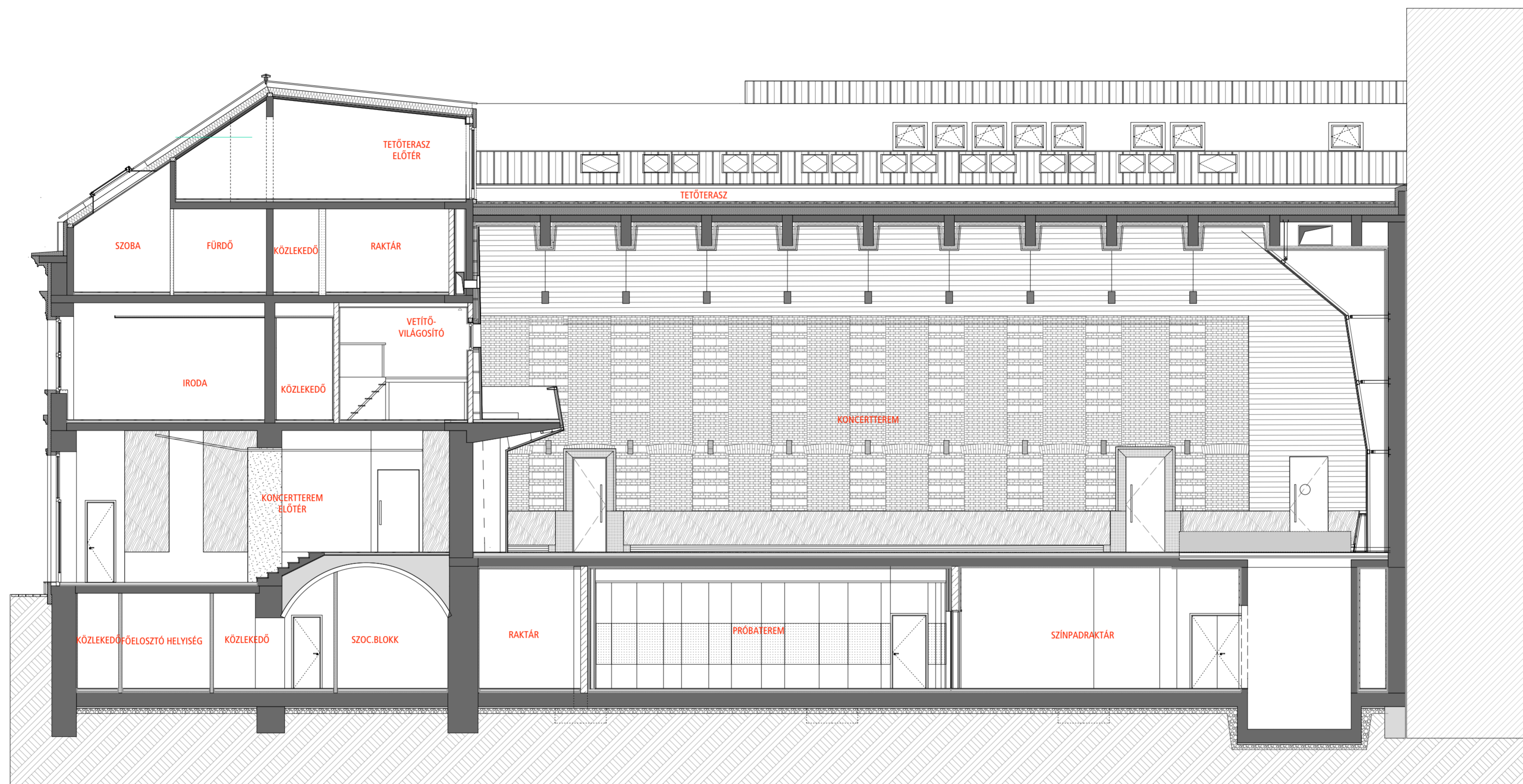
C-C METSZET
