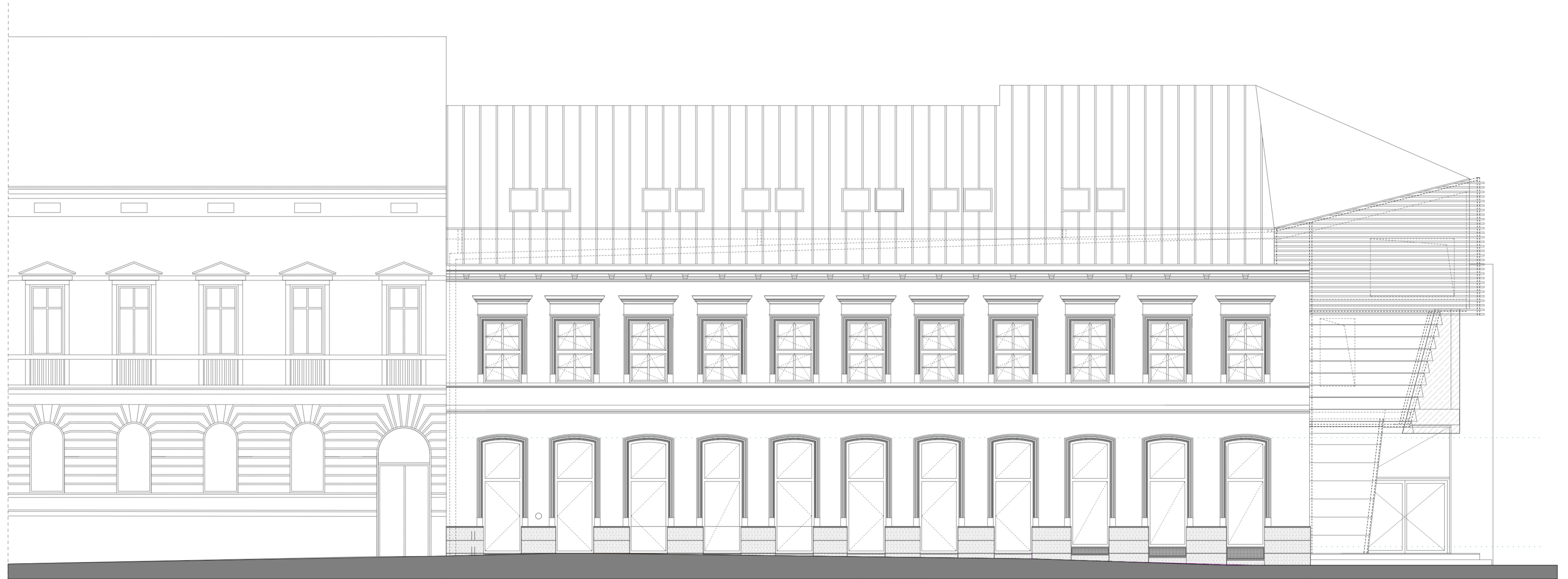
IMRE UTCAI HOMLOKZAT
