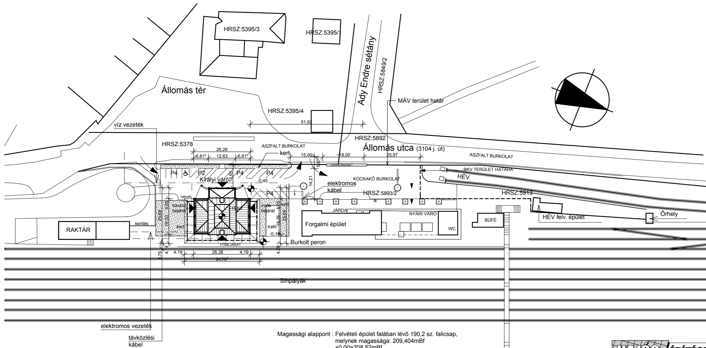
HELYSZÍNRAJZ M=1:1000
