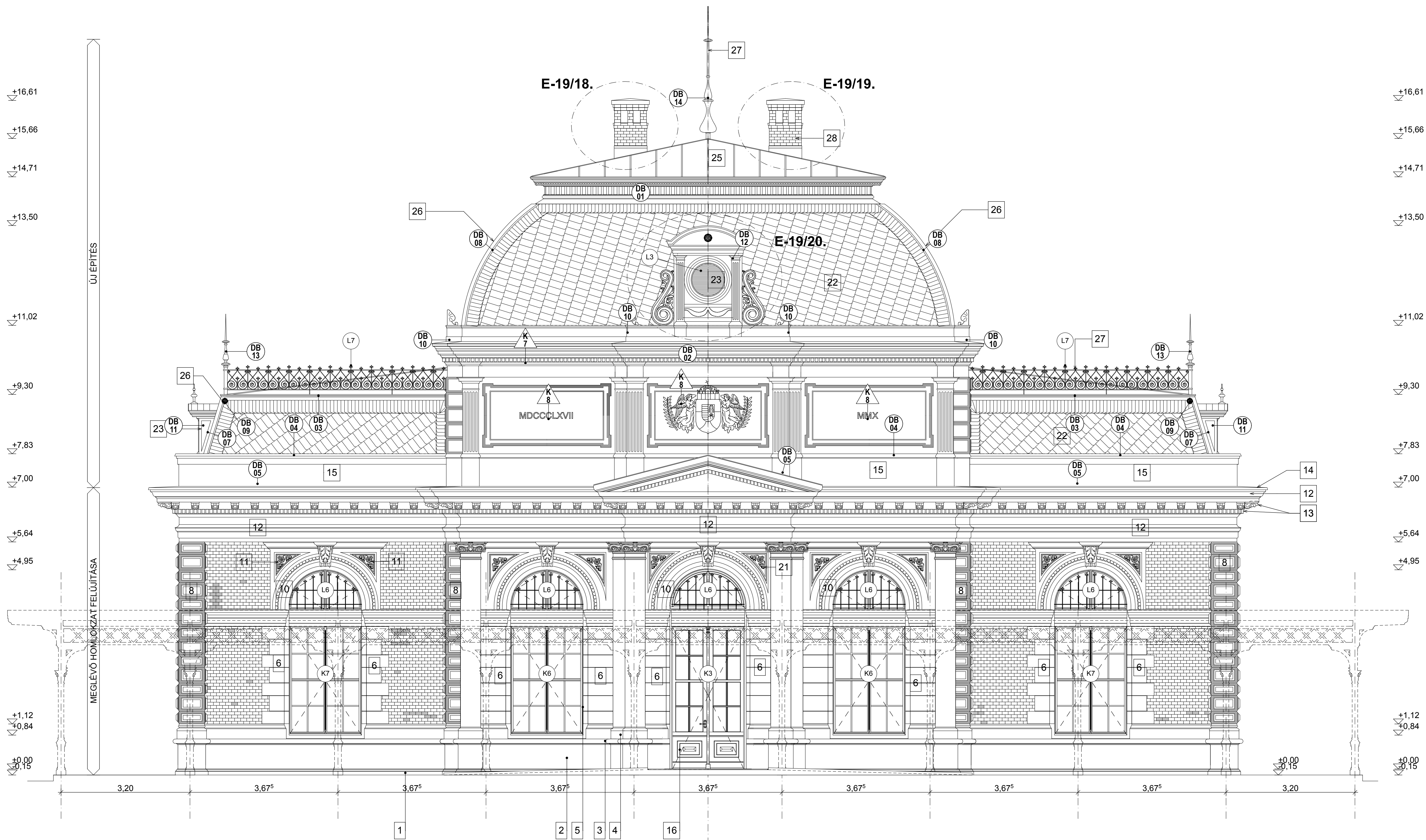
KELETI HOMLOKZAT M=1:50
