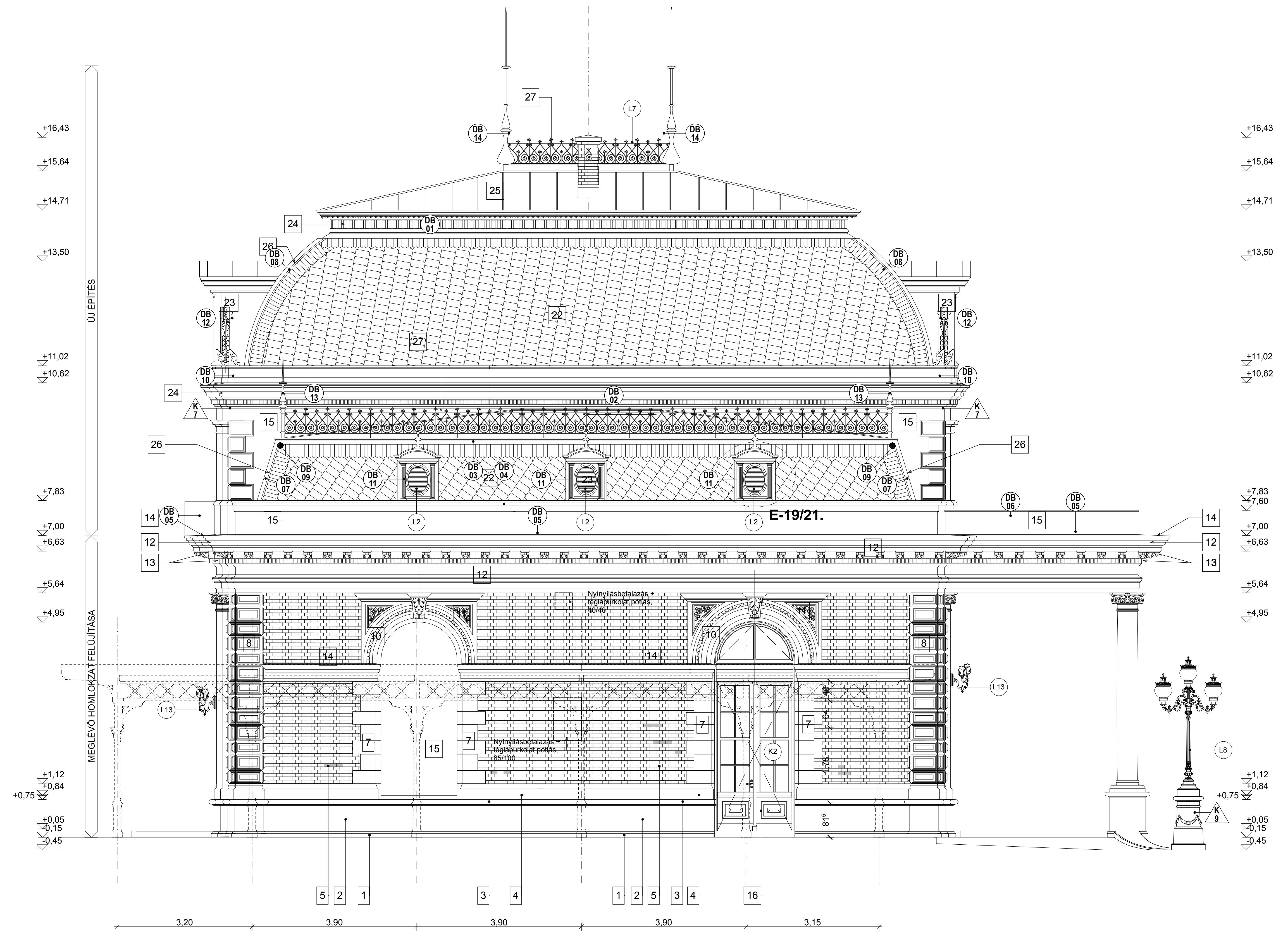
ÉSZAKI HOMLOKZAT M=1:50
