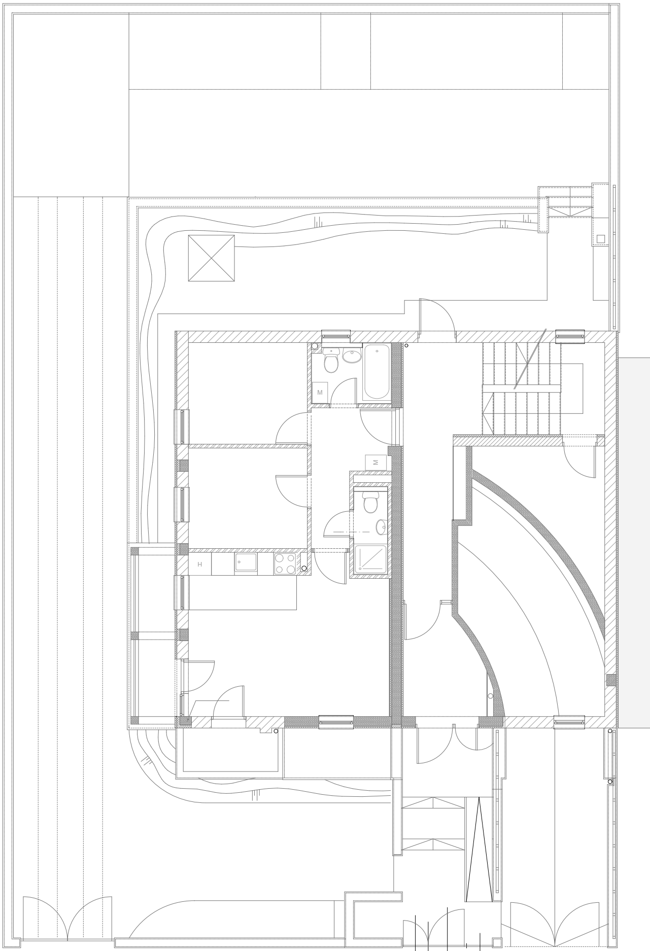
Földszinti alaprajz
