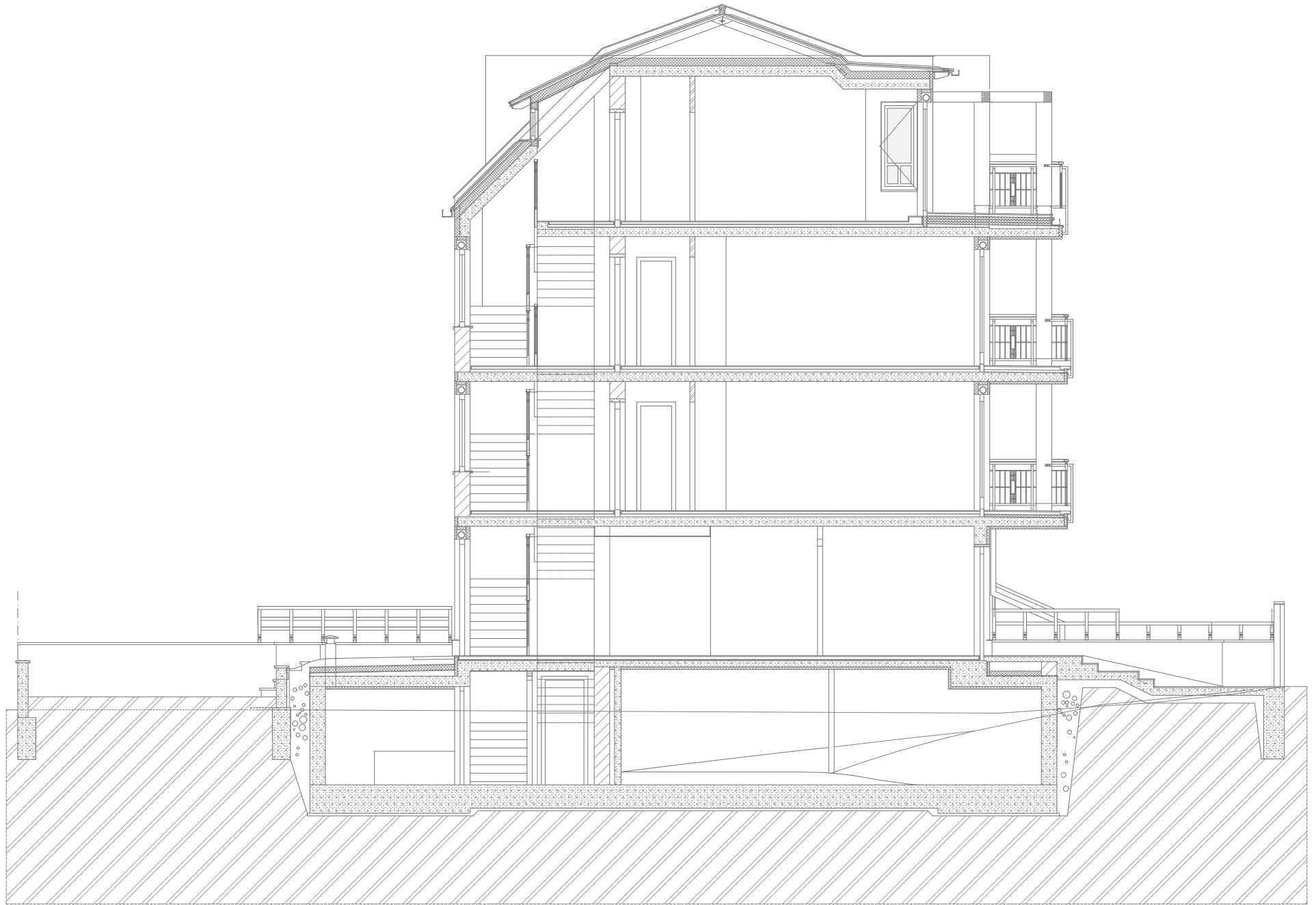
keresztmetszet
