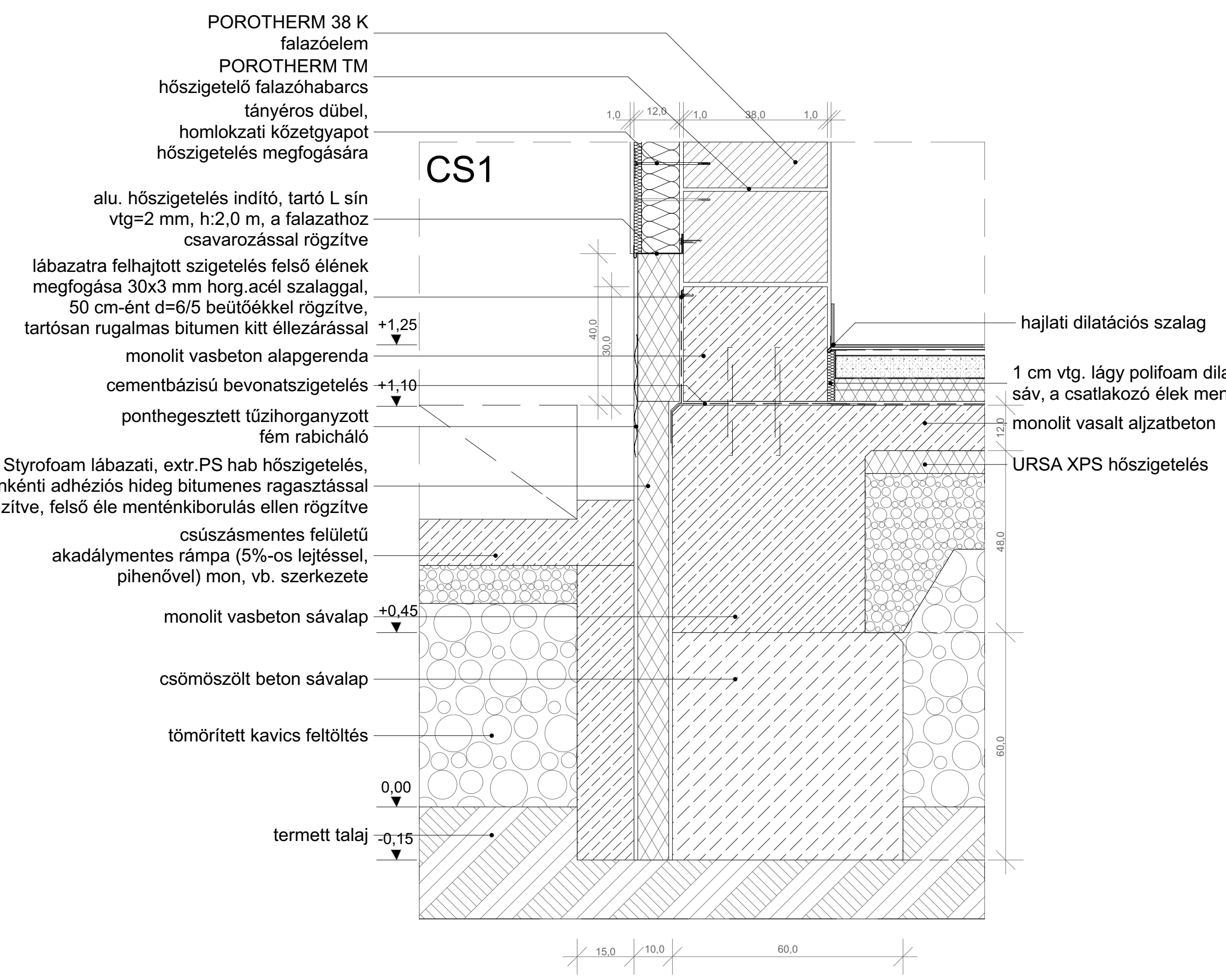
SZERKEZETI VÁZLATOK
