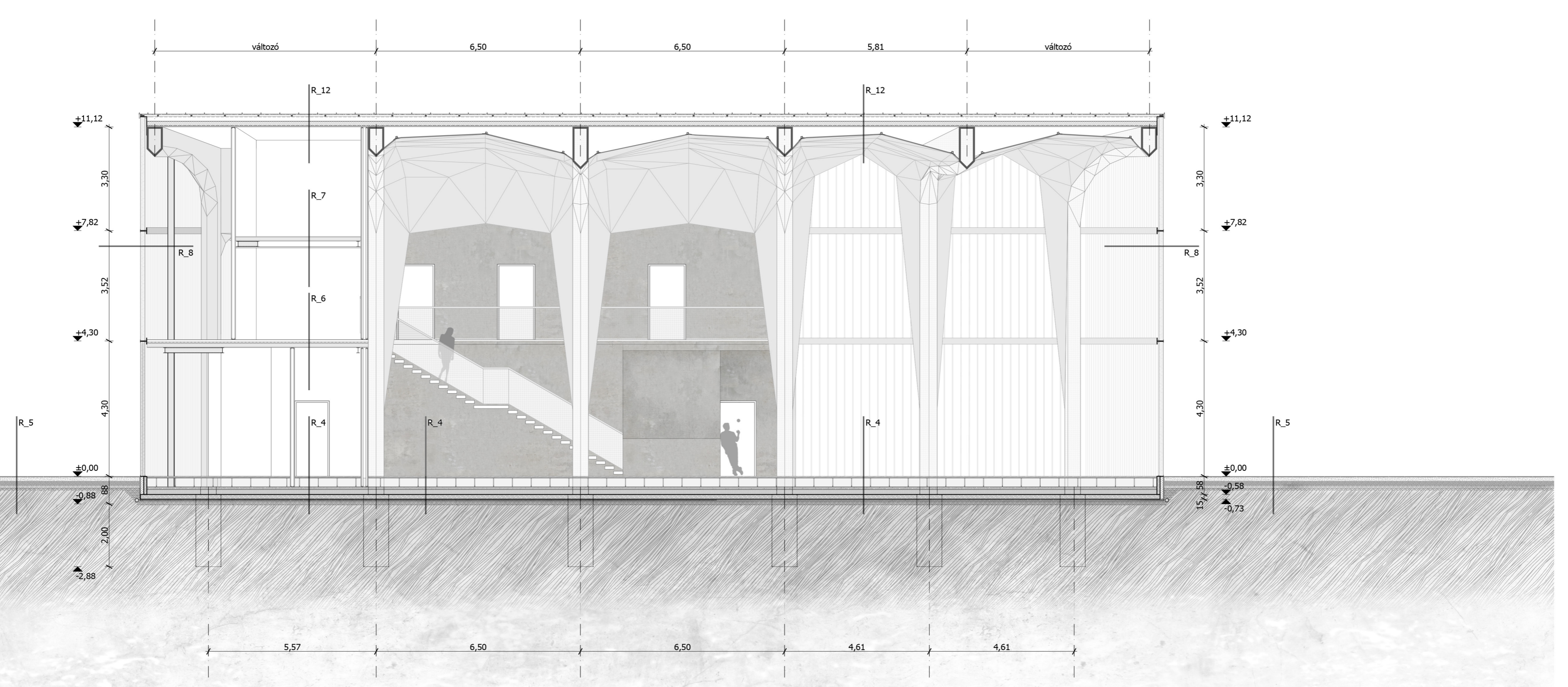
b b metszet m=1:100
