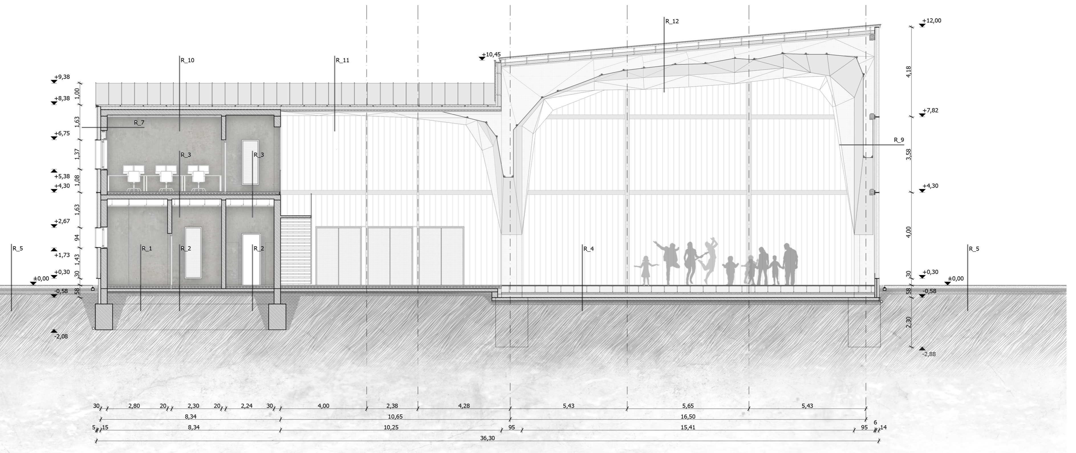
a a metszet m=1:100
