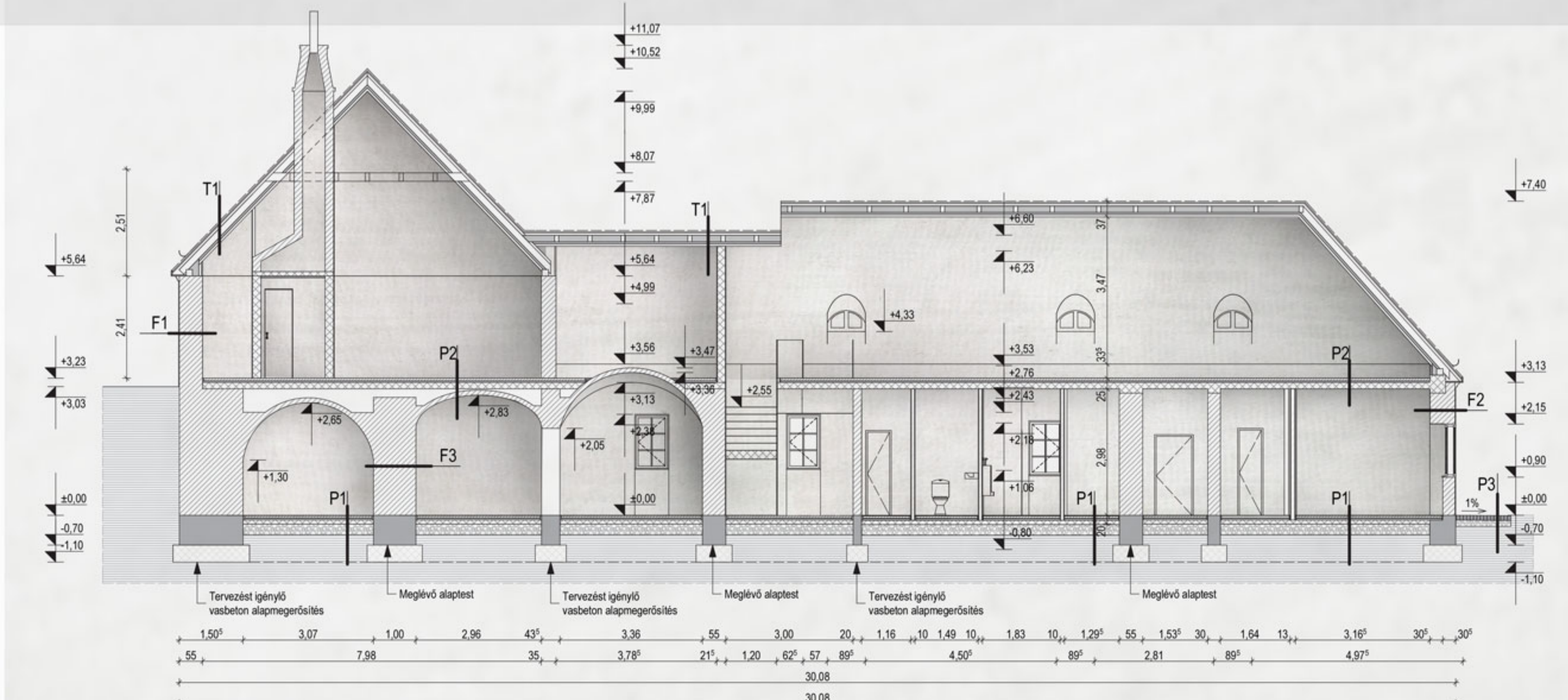
KŐFARAGÓ HÁZ _ B-B METSZET _ M=1:100
