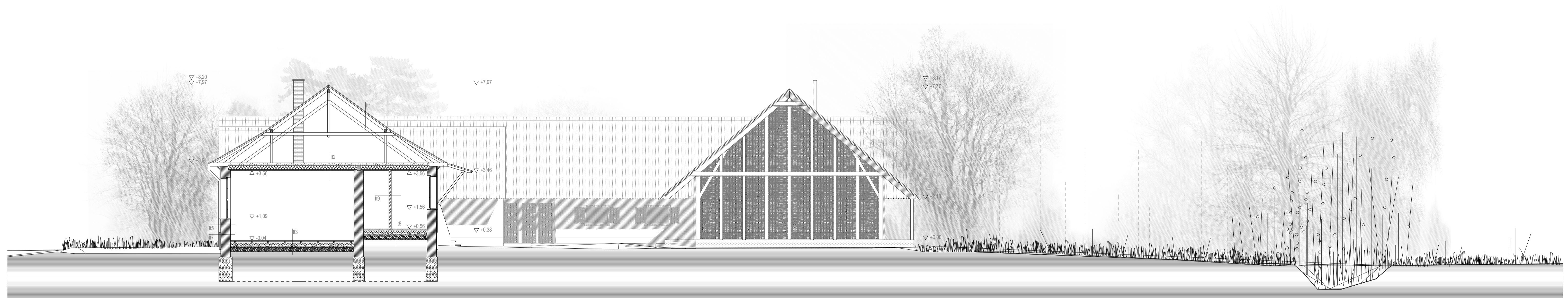
B-B KERESZTMETSZET
