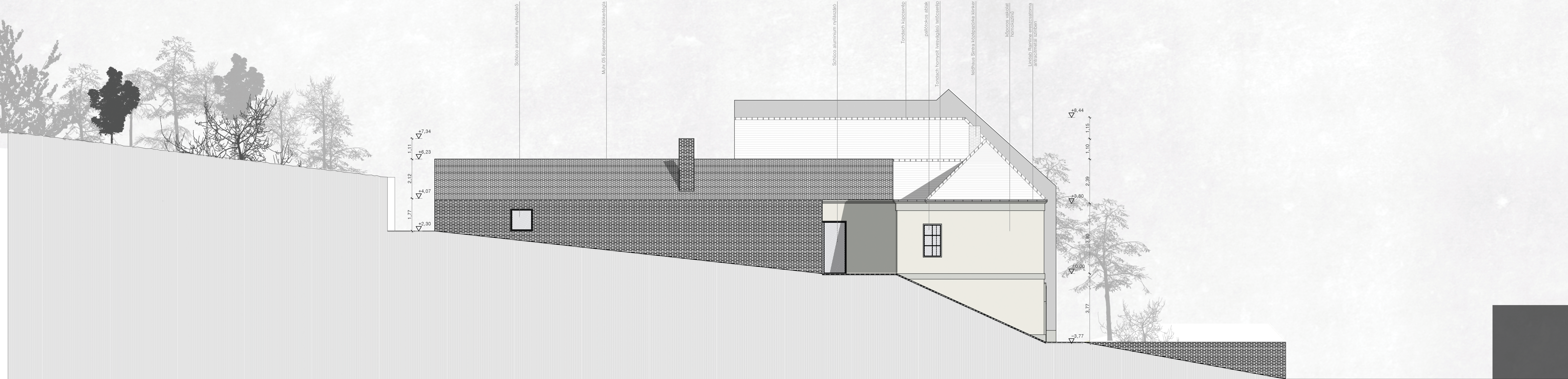
déli homlokzat 1:100
