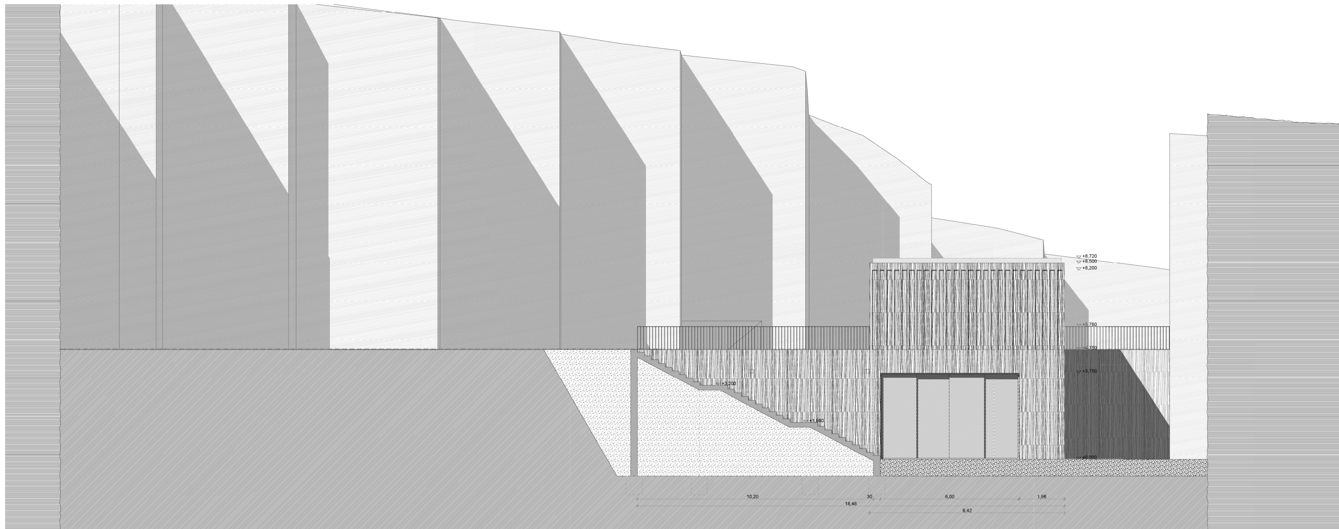
Kéleti homlokzat és metszet a hasitékot az udvarral összekötő lépcsőn keresztül
