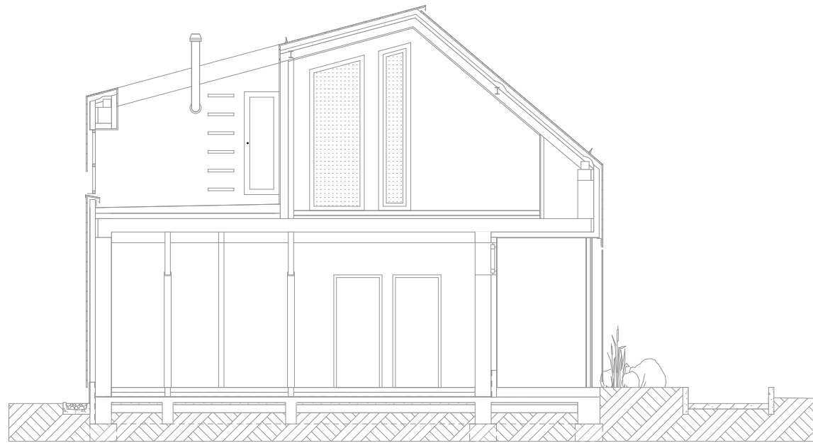
A-A METSZET
